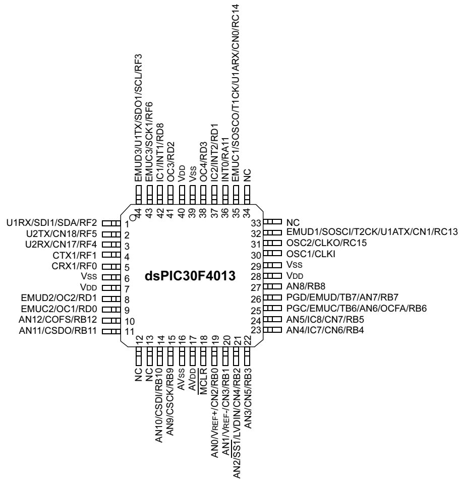
44-Pin TQFP
