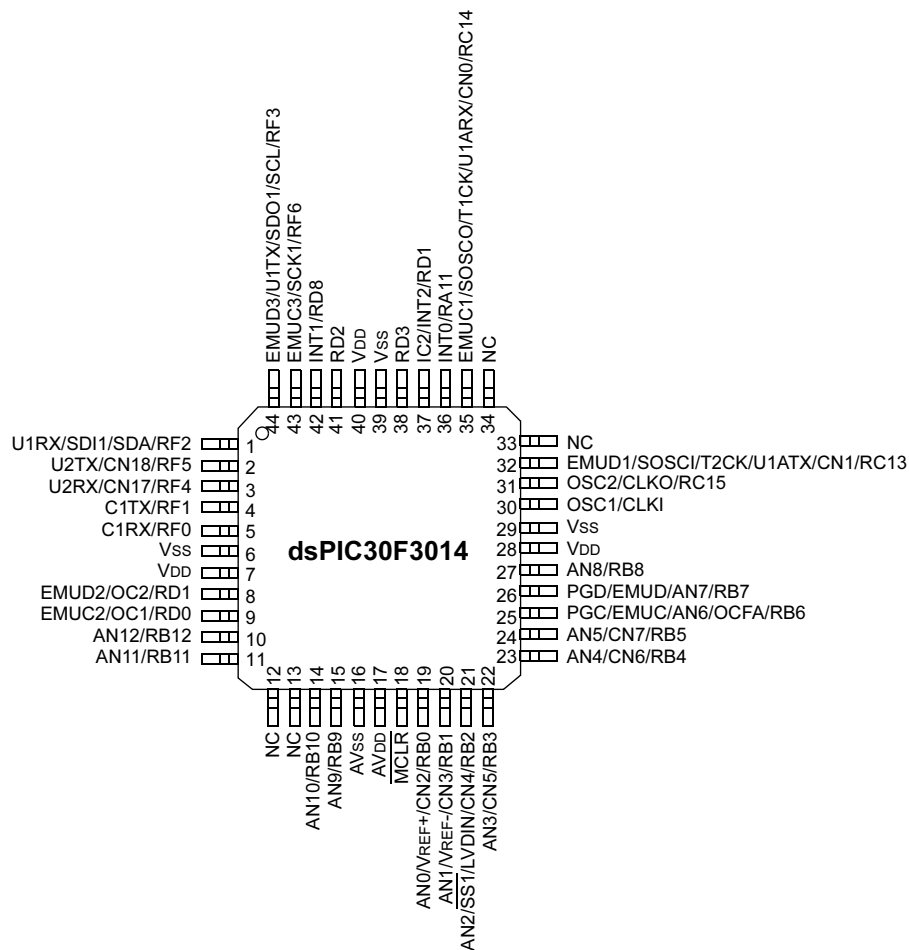
44-Pin TQFP
