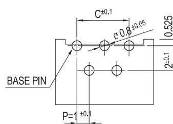
P.C.B. LAY-OUT(B-TYPE)
