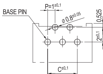
P.C.B. LAY-OUT(A-TYPE)
