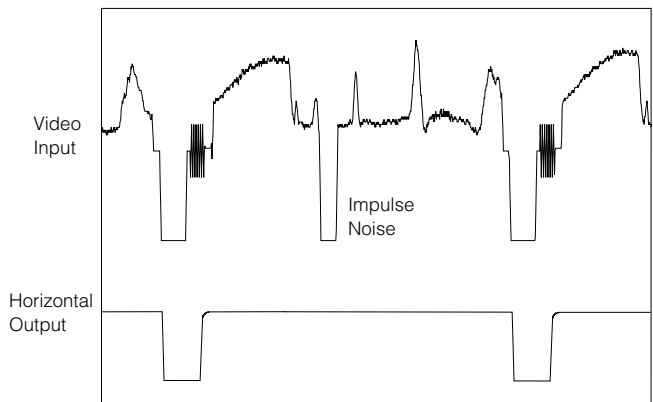
Fig. 16 Horizontal Output
