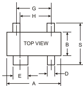
SOT-343 / SOT-143
