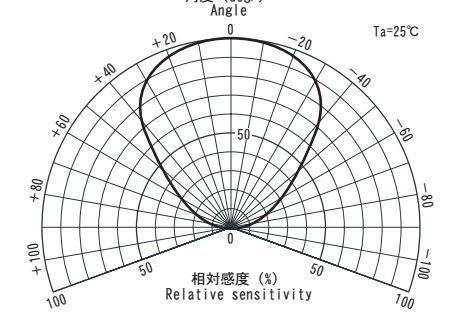
■指向特性
