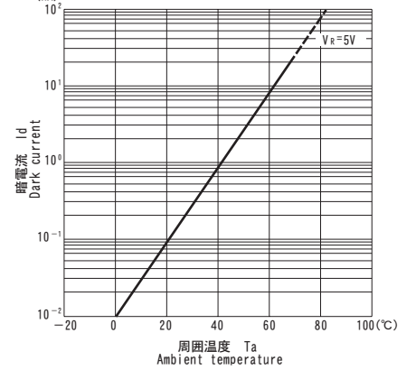
■ 暗電流/周囲温度特性 I_d/T_a
