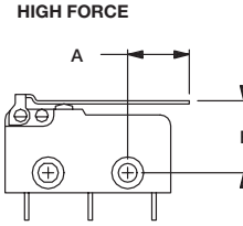
FIG. 3 Lever
