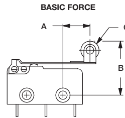
FIG. 7 Lever Roller
