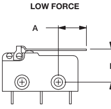
FIG. 4 Lever
