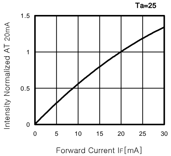
Fig. 2 Iv-IF
