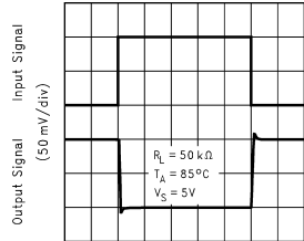
Time (10 \mu s /div) DS100979-D8
