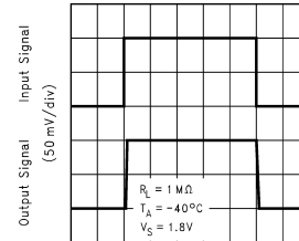
Time (10 \mu s /div) DS100979-E7
