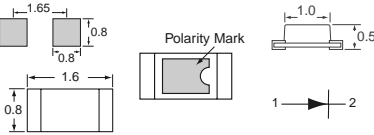
Fig. 3 — 0603 (1608) Leadless-TSS Type
