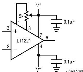
Offset Nulling
