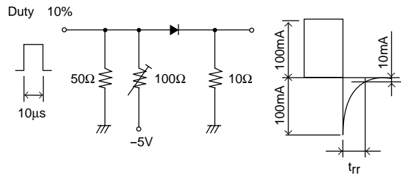
trr 指定回路図 (SBD 部)
