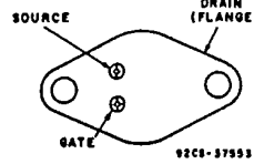
JEDEC TO-204AA
