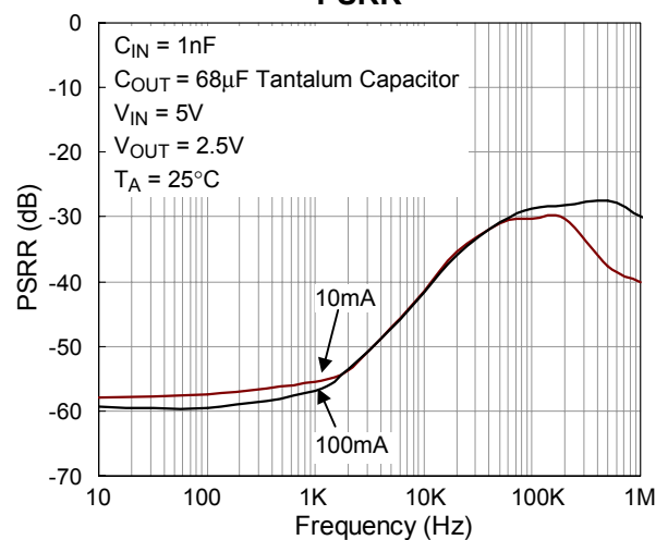
PSRR
