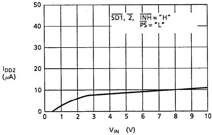
4-4-1 I_{DD2} - V_{IN}
