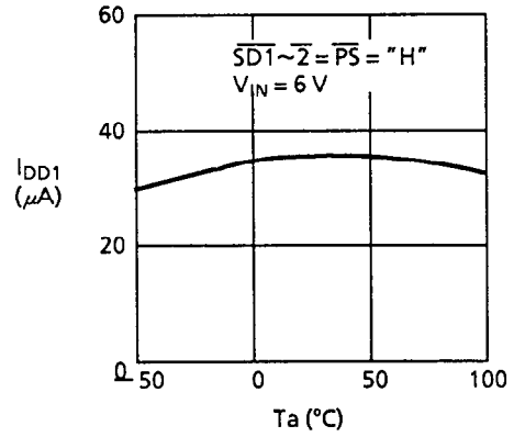
4-3-2 I_{DD1} - Temperature
