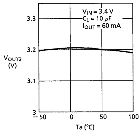
1-1-6 V_{OUT3} -Temperature
