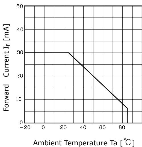
Fig. 3 I_F - T_a
