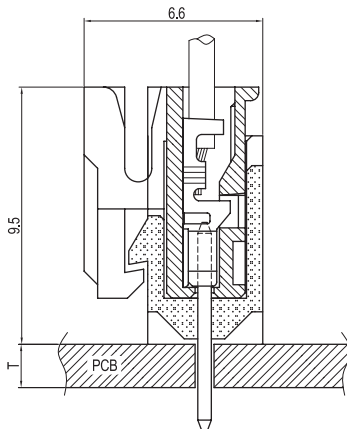
PCB ASS'Y
