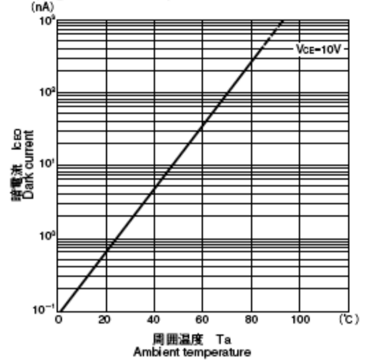
■暗電流/周囲温度特性 I_{CE0}/T_a
