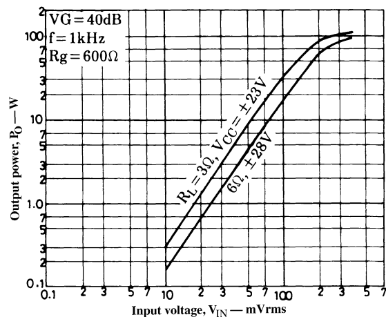
P_O - V_{IN}
