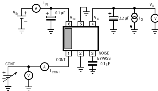
SOT-23L
