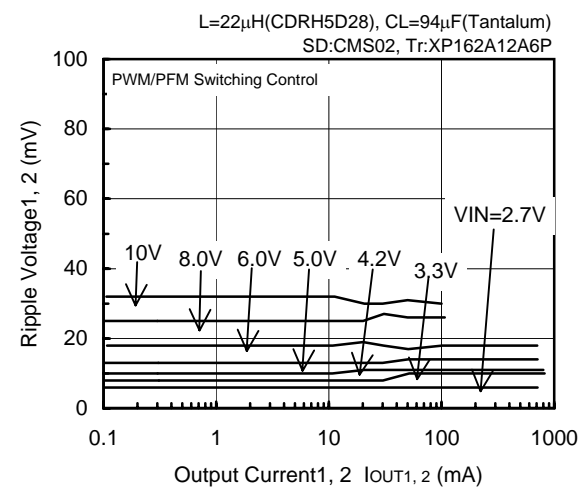
FOSC=300kHz, VOUT1, 2=2.5V
