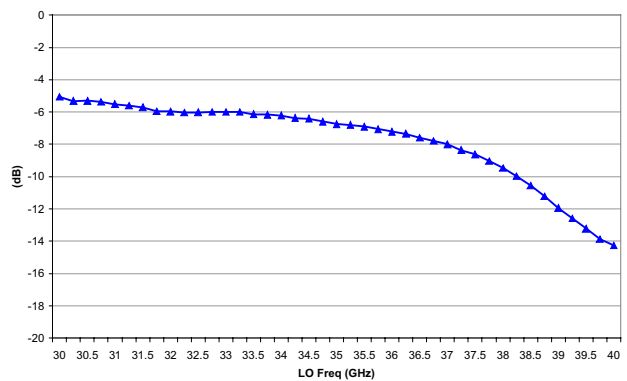
LO Return Loss (dB)
