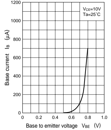
I_B - V_{BE}
