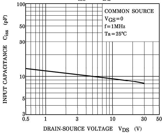
C_{iss} - V_{DS}
