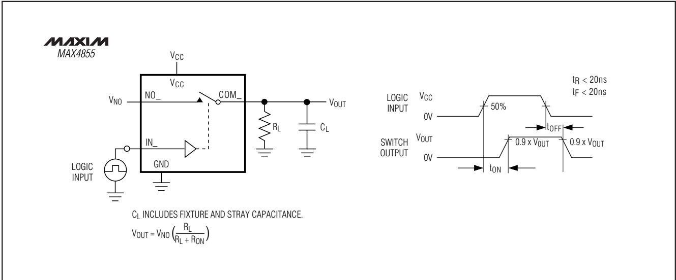
图 1. 开关时间
