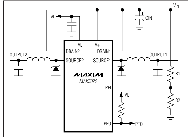
图5. Dying Gasp电路监视输入电源
