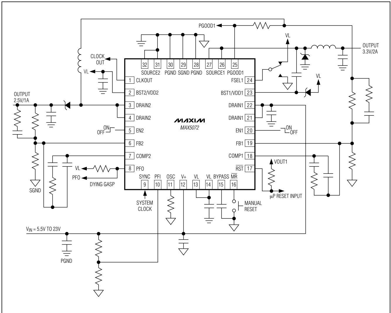
图9. 降压型 - 升压型应用
