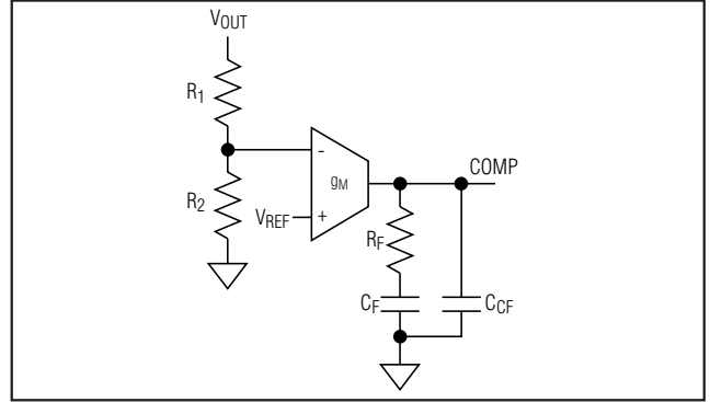
图7. II型补偿网络
