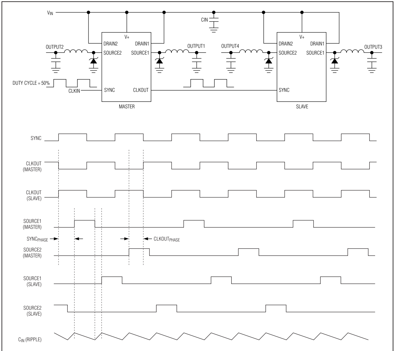
图3. 同步控制器
