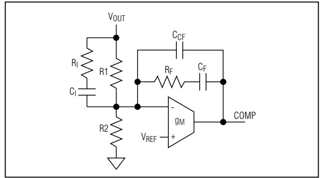
图8. III型补偿网络
