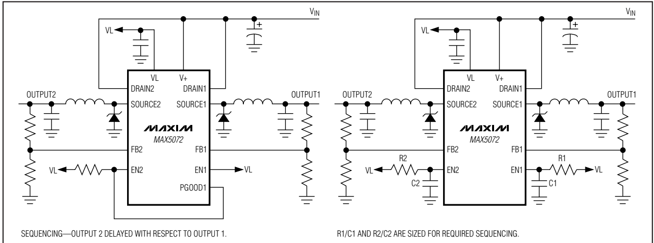
图4. 电源排序配置
