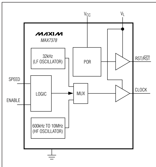
图 1. 功能框图
