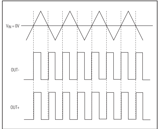
图1. 无输入信号时MAX9704的输出
