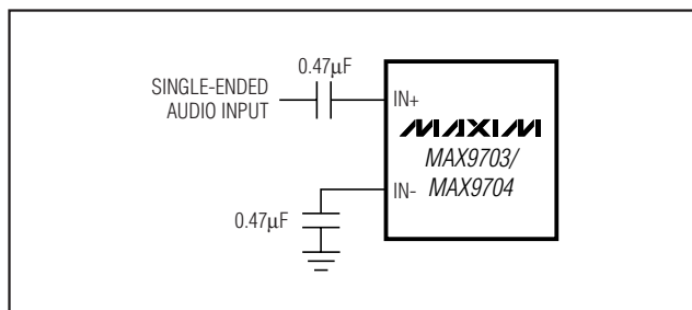
图4. 单端输入
