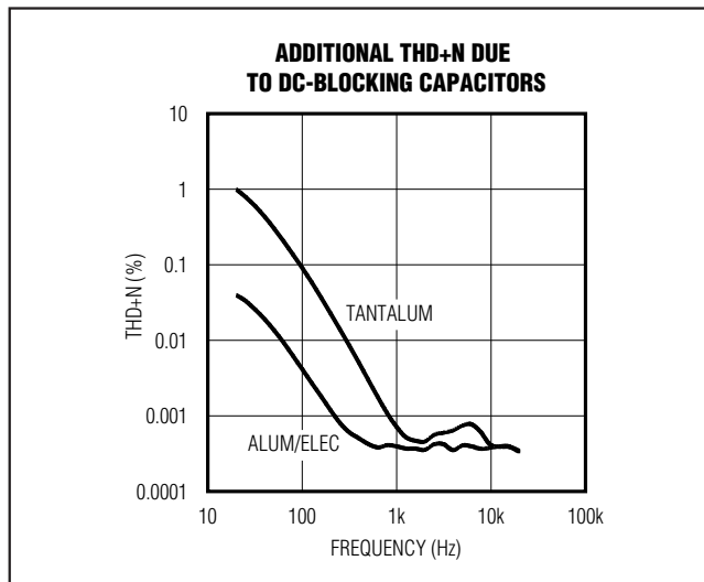
图5. 隔直电容引起的失真
