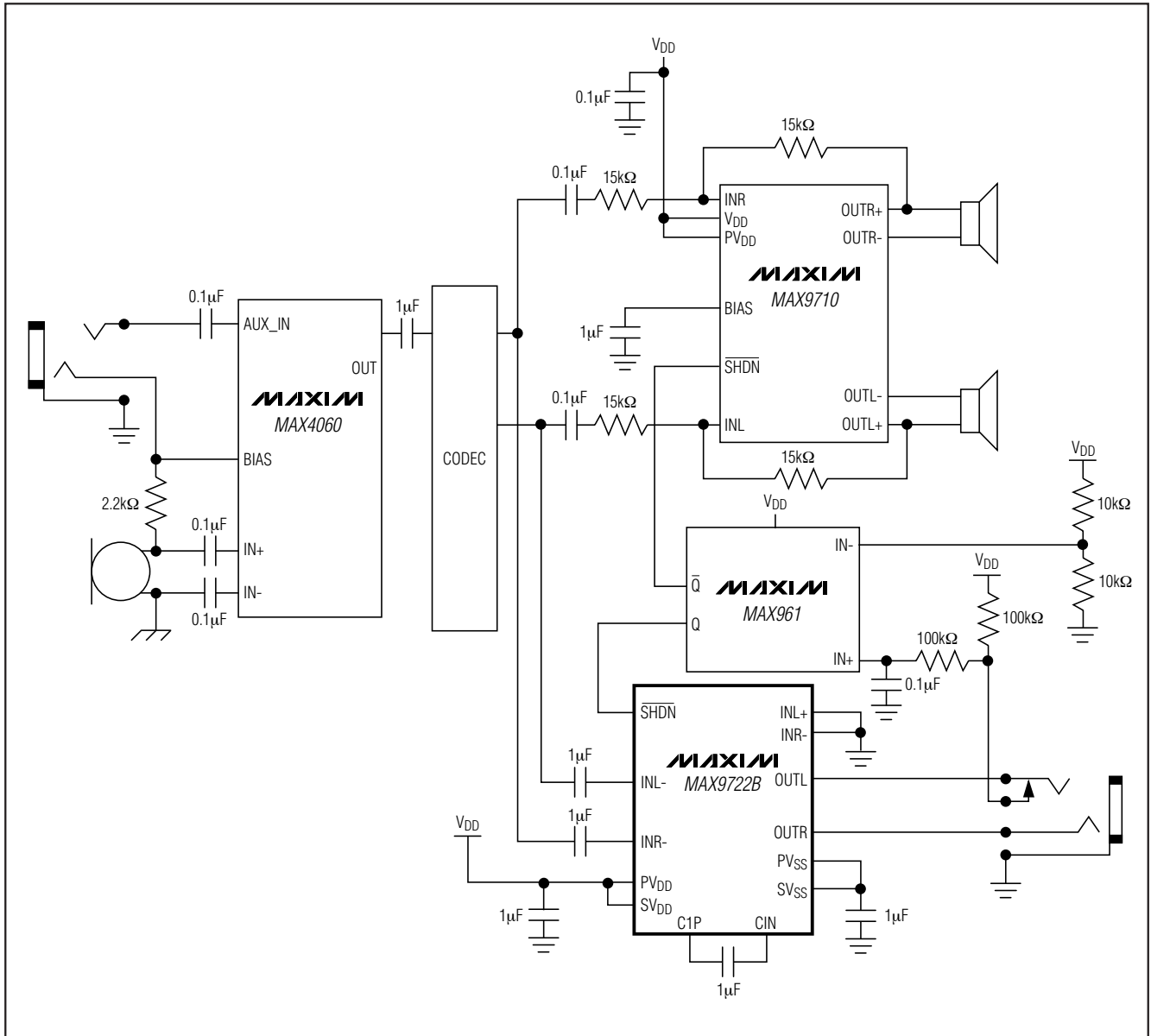
系统框图
