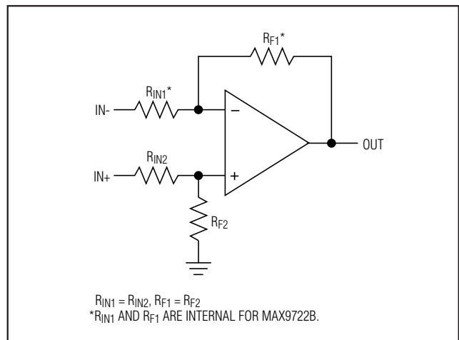
图 2. 差分输入配置
