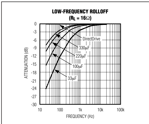
图4. 普通隔直电容的低频衰减
