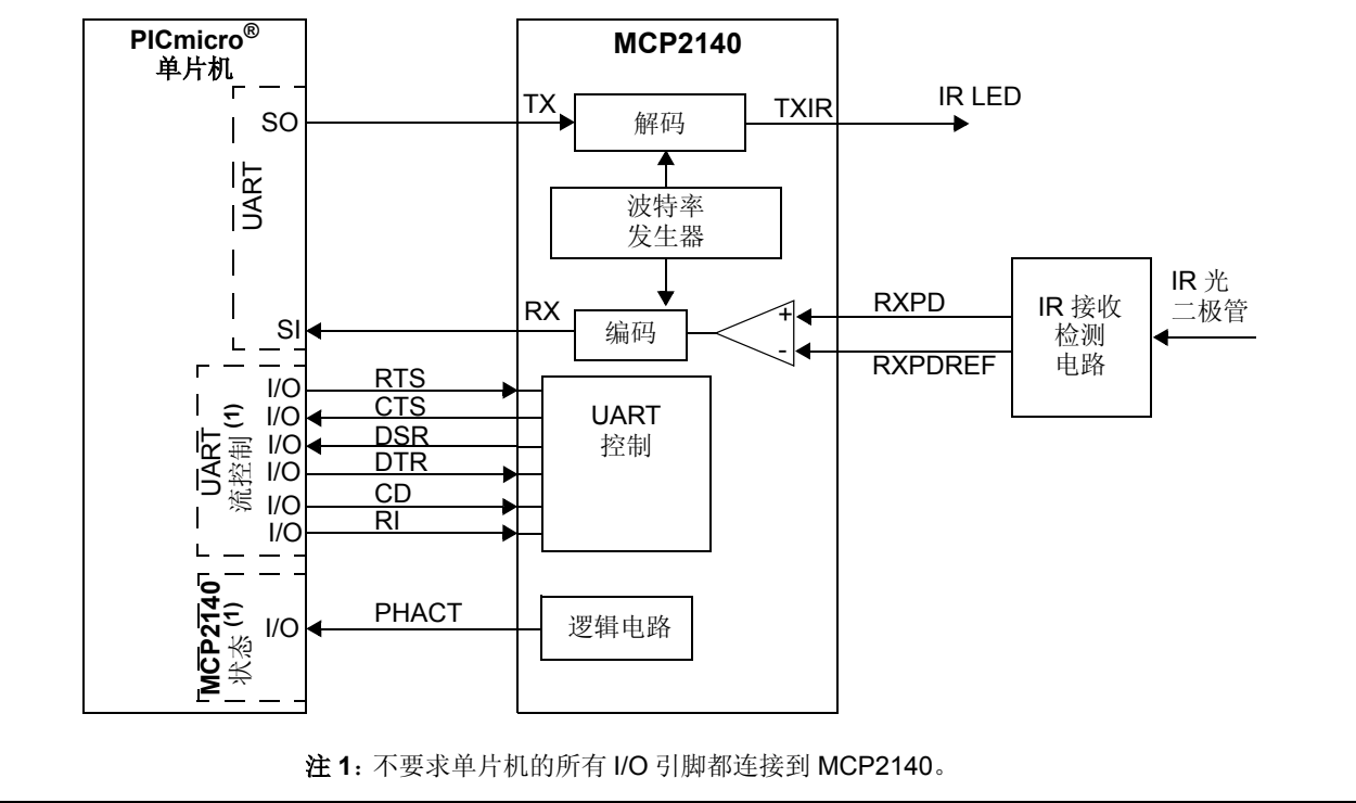
图 1-1: 系统框图
