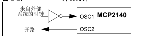
图 2-2: 外部时钟
