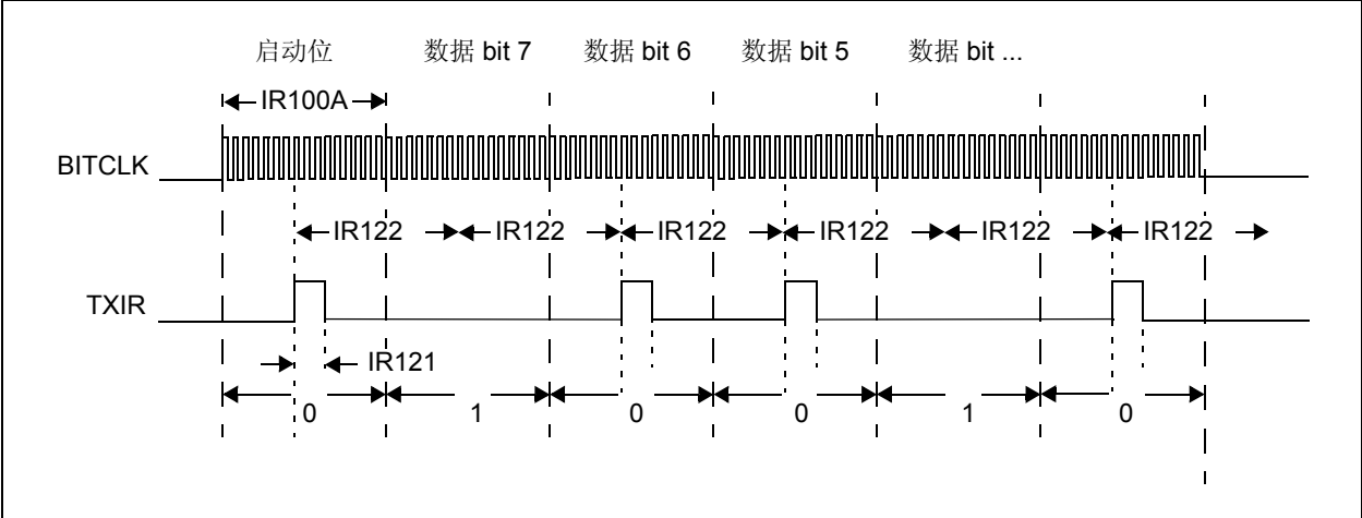
图 4-8: TXIR 波形
