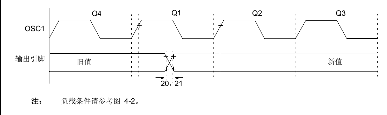
图 4-4：输出波形
