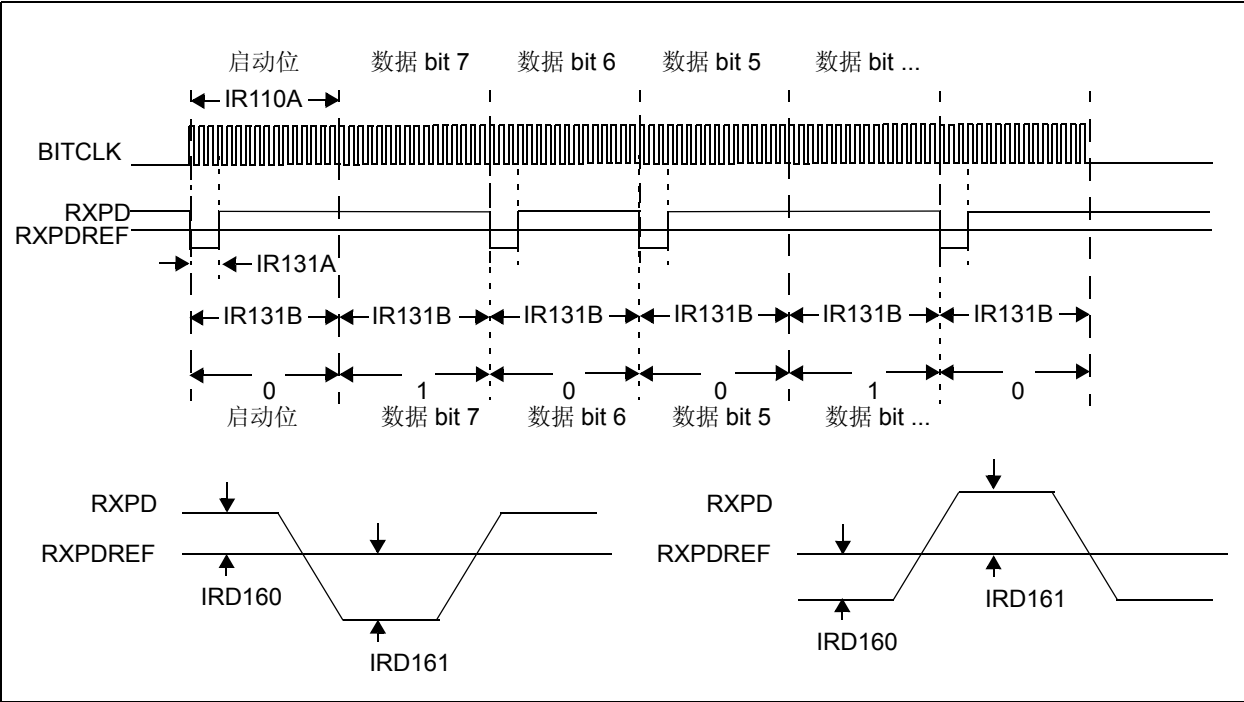
图 4-9: RXPД/RXPДREF 波形
