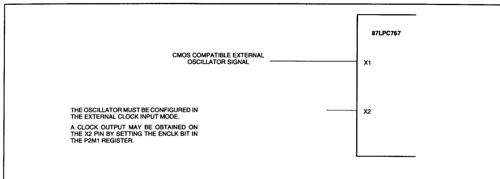
图 18 使用外部时钟输入
