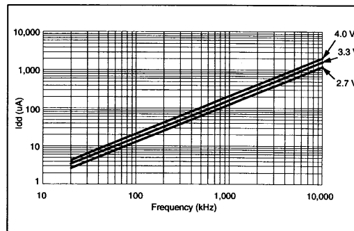
图 45 典型的空闲 Idd 对应频率(外部时钟, 25°C, LPEP=1)
