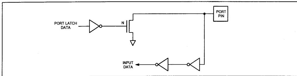
图 12 开漏输出
