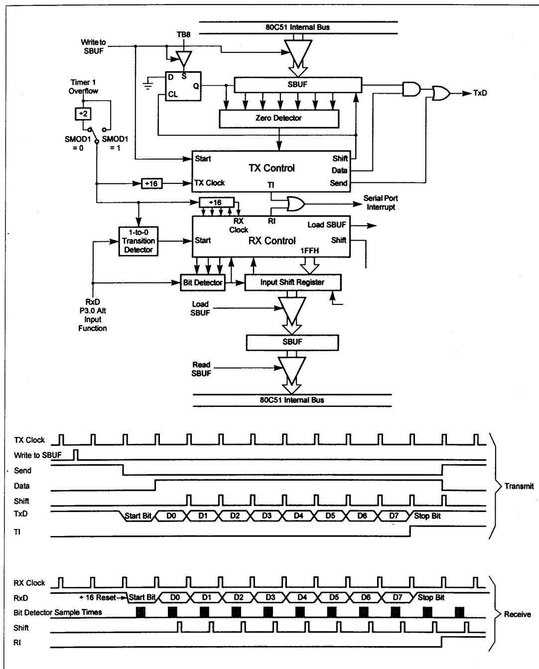
图 31 串口模式 1
