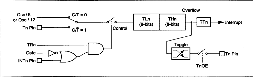
图 26 模式 1 方式时定时/计数器 0 或 1 (16 位计数器)
