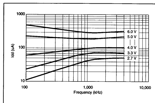
图 43 典型的中频振荡器 Idd(25°C)
