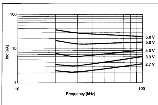
图 42 典型的低频振荡器 Idd(25°C)
