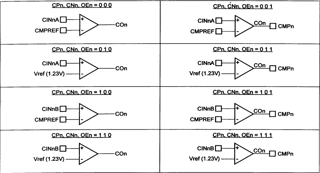
图 6 比较器配置
