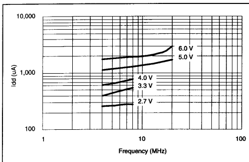
图 44 典型的高频振荡器 Idd(25°C)
