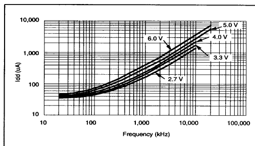
图 47 典型的空闲中 Idd 与对应频率(外部时钟, 25°C, LPEP=0)
