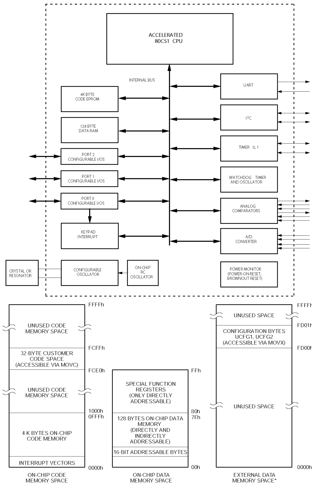
图 1 P87LPC767 程序和数据存储器分布图
