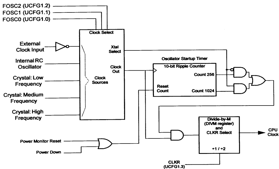
图 18 使用外部时钟输入
