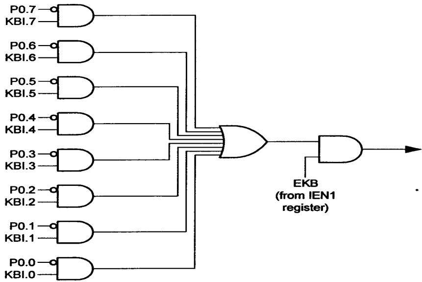
图 15 键盘中断
