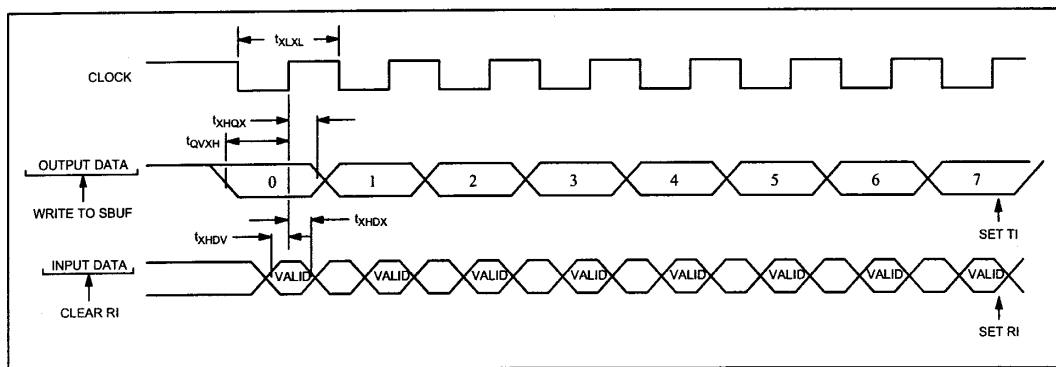
图 40 移位寄存器模式时序
