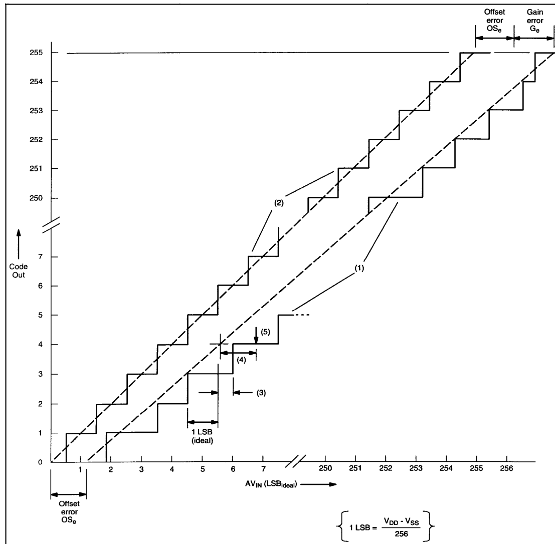
图 39 A/D 转换特性
