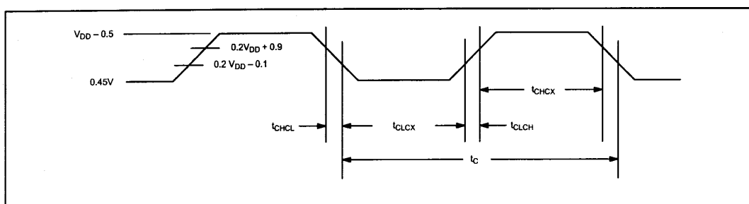
图 41 外部时钟时序
