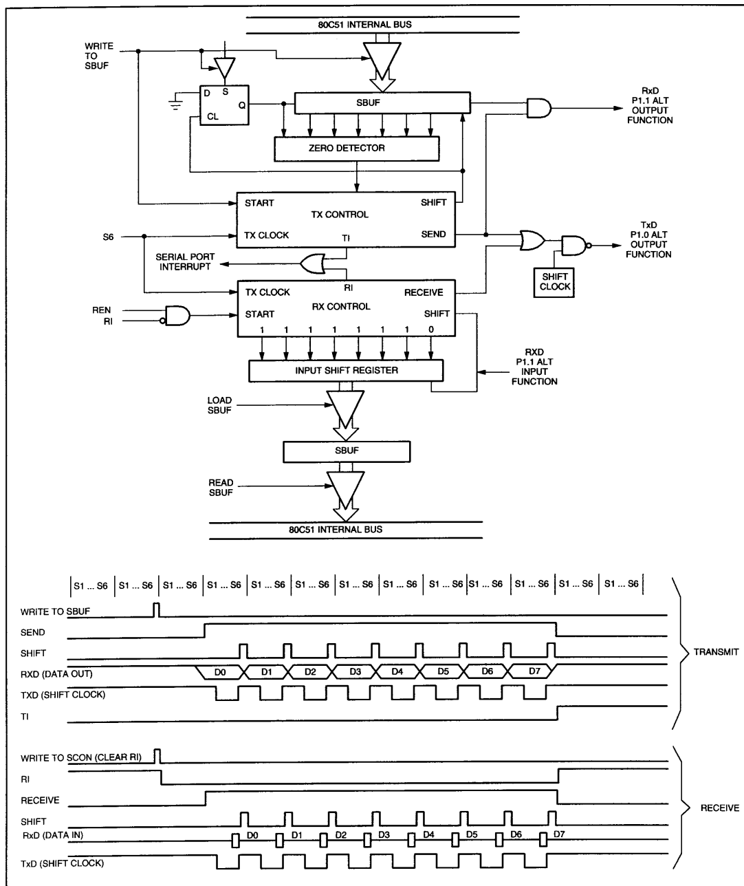
图 30 串口模式 0
