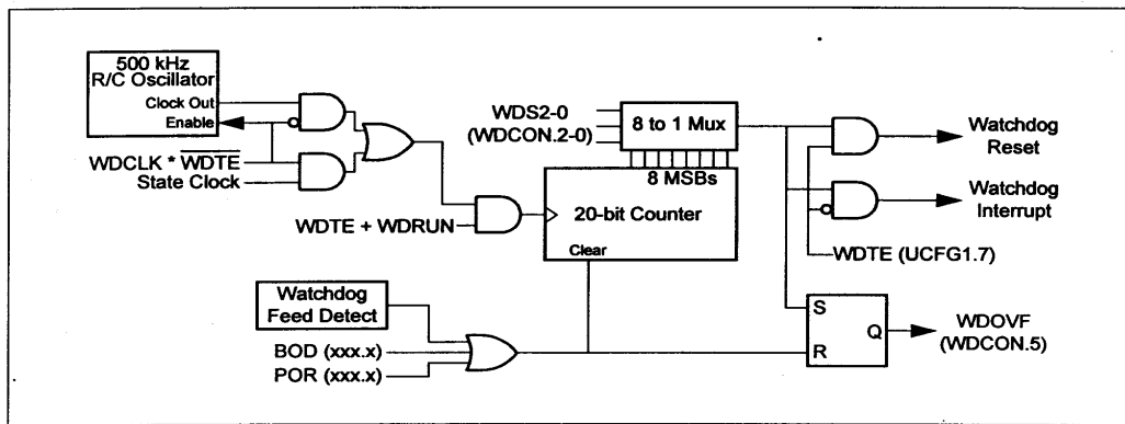
图 34 看门狗定时器
