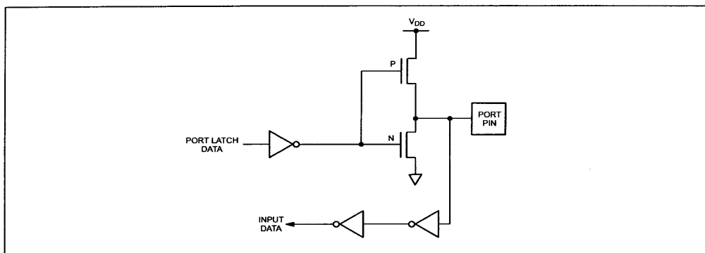
图 13 上拉输出
