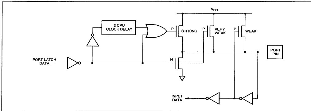
图 11 准双向口输出
