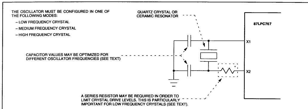
图 17 晶振的使用
