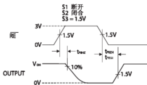
图 12 接收器使能和禁能波形
