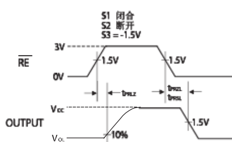
图 12 接收器使能和禁能波形
