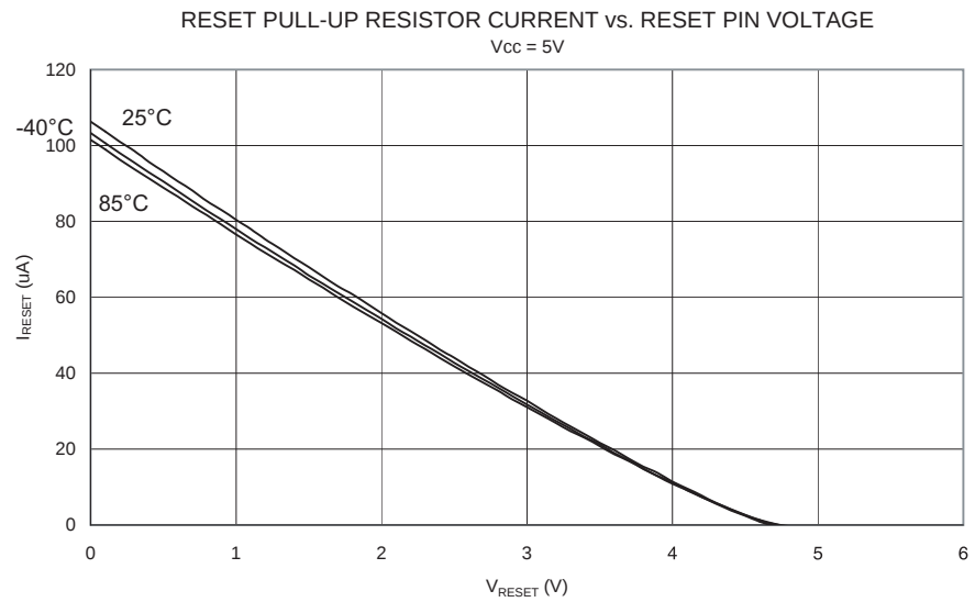
Figure 175. 复位 (Reset) 引脚上拉电阻电流和 Reset 引脚电压的关系 ( V_{CC} = 5V )
