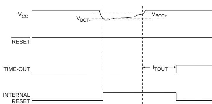
Figure 19. 工作过程中发生掉电检测复位
