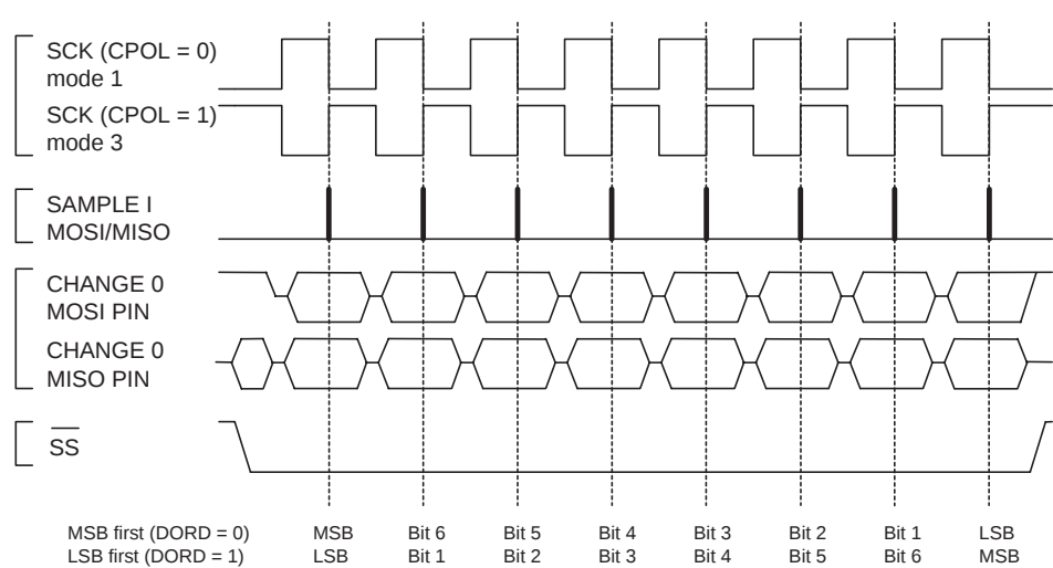
Figure 68. CPHA = 1 时 SPI 的传输格式
