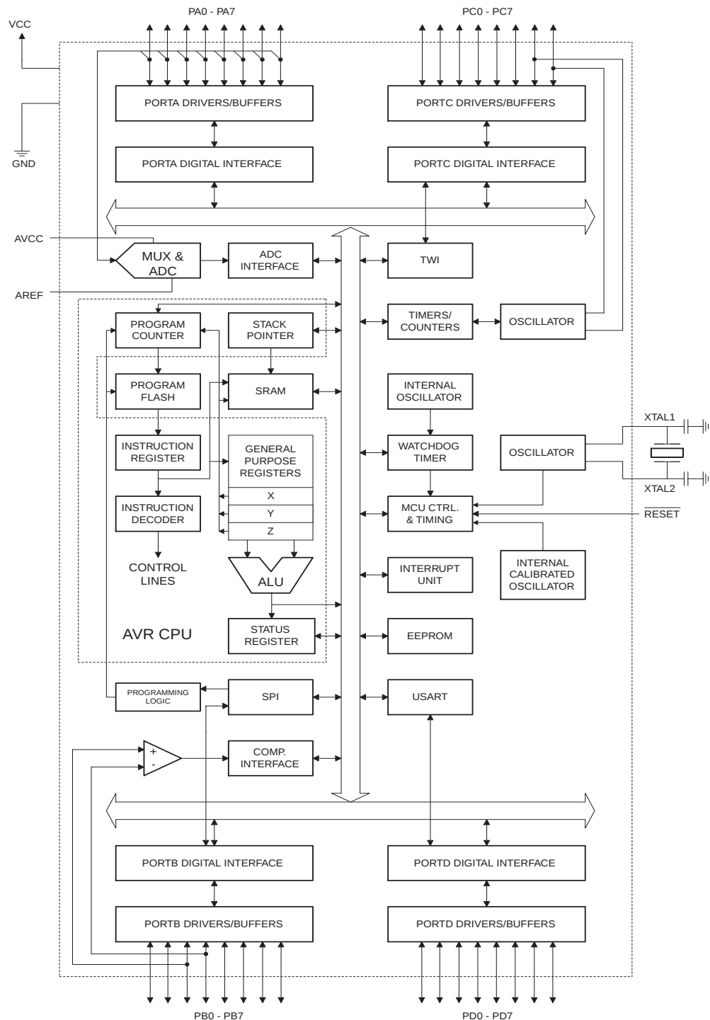
Figure 2. 结构框图
