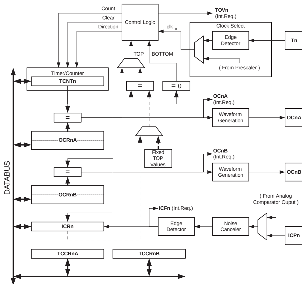
Figure 40. 16 位 T/C 框图 (1)
