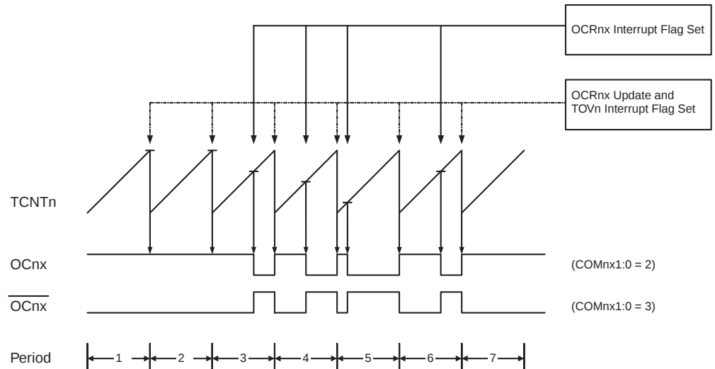
Figure 59. 快速 PWM 模式时序图
