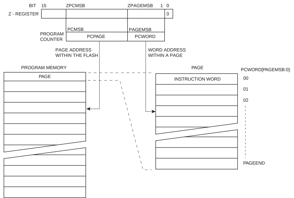
Figure 118. SPM (1) 的寻址
