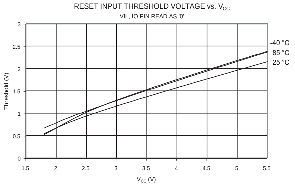
Figure 164. Reset 输入门限电压和 V_{CC} 的关系 ( V_{IL} , Reset 引脚读值为 “0”)
