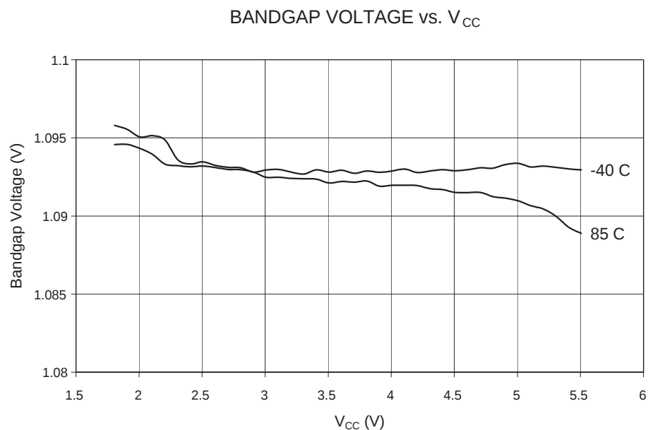
Figure 169. 能隙电压和 V_{CC} 的关系
