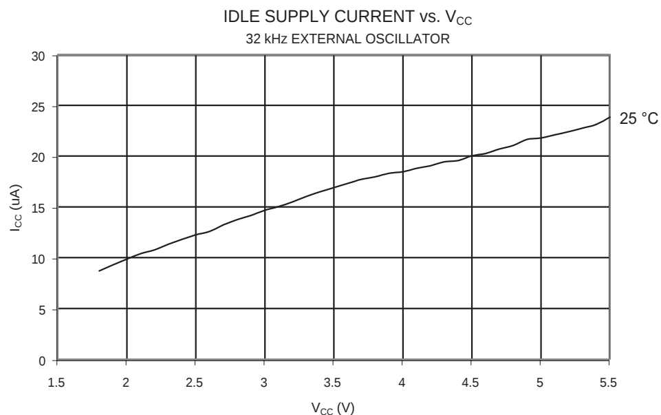
Figure 145. 空闲模式电流和 V_{CC} 的关系 (32 kHz 外部晶振)
