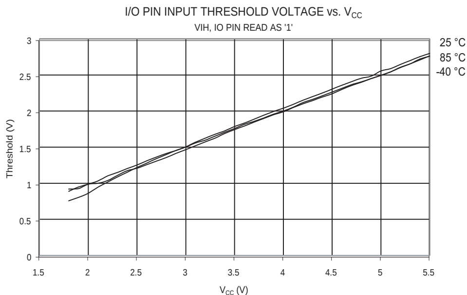
Figure 161. I/O 引脚输入门限电压和 V_{CC} 的关系 ( V_{IH} , I/O 引脚读值为“1”)
