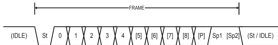
Figure 73. 帧格式
