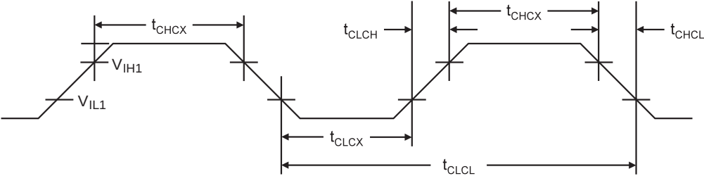
Figure 130. 外部时钟波形
