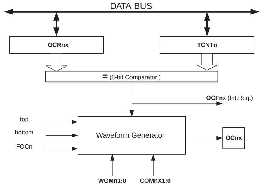
Figure 56. 输出比较单元方框图
