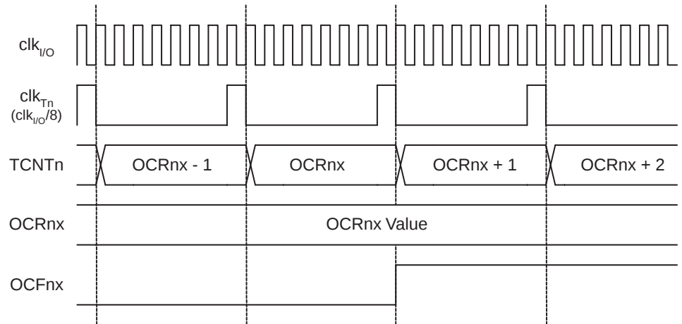
Figure 51. T/C 时序图，置位 OCF1x，预分频器为 f_{\text{clk\_I/O}}/8
