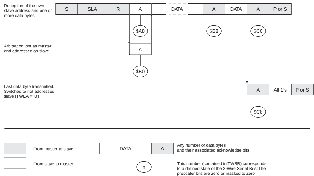
Figure 96. 从机发送模式的格式和状态
