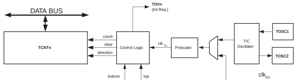
Figure 55. 计数器单元方框图
