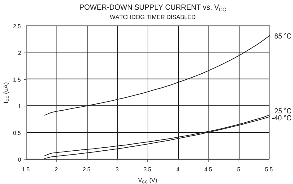
Figure 146. 掉电模式电流和 V_{CC} 的关系 (看门狗定时器禁用)
