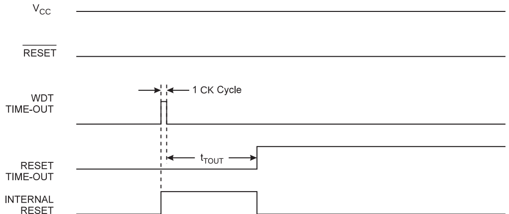
Figure 21. 工作过程中发生看门狗复位
