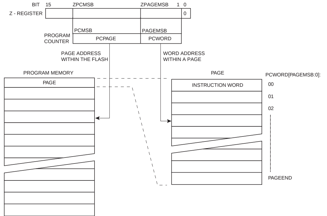
Figure 115. SPM (1) 的寻址
