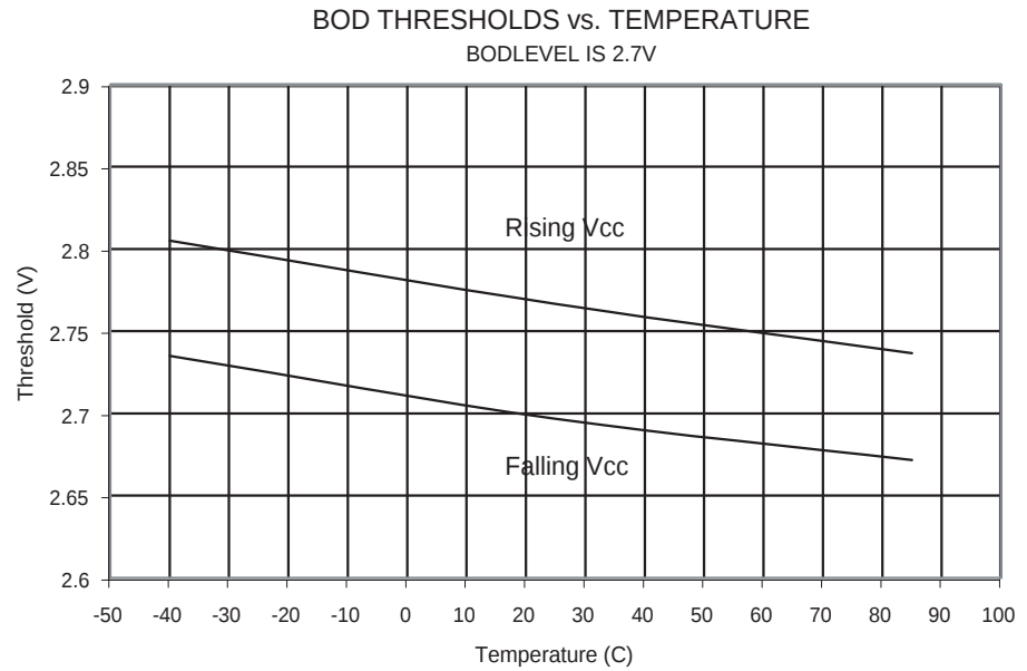
Figure 167. BOD 门限值和温度的关系 (BOD 电平为 2.7V)
