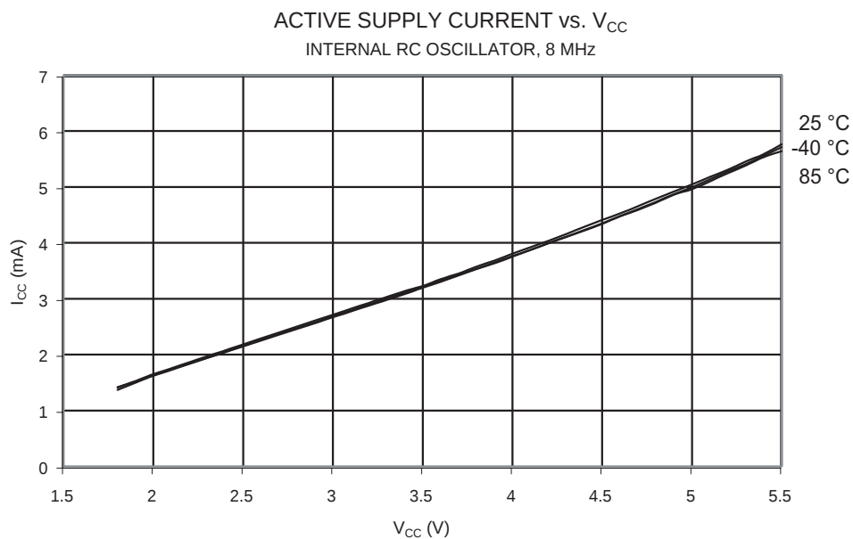
Figure 138. 工作电流和 V_{CC} 的关系 (内部 RC 振荡器, 8 MHz)
