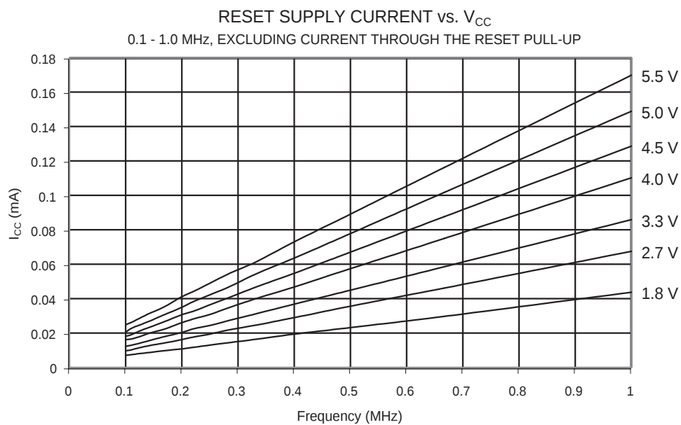
Figure 178. 复位电流和 V_{CC} 的关系 (0.1 - 1.0 MHz，包括流经复位上拉电阻的电流)
