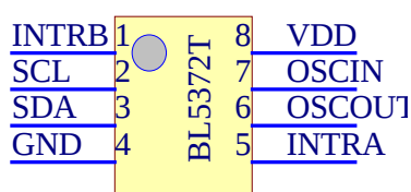
8 脚 TSSOP
