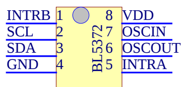
8 脚 SOP
