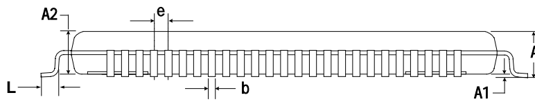
图 4.2 TQFP-100 封装图
