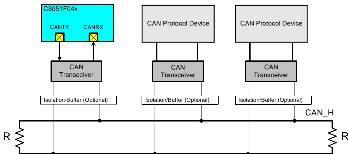
图 18.1 典型 CAN 总线配置
