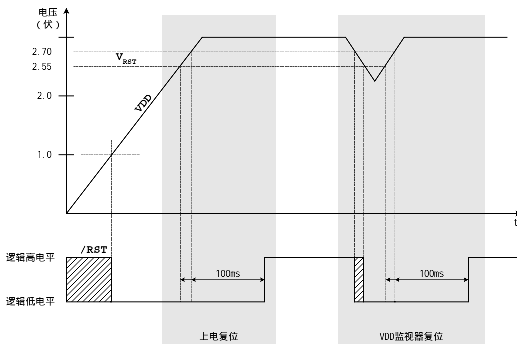
图 13.2 复位时序图
