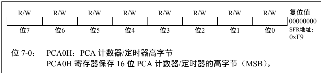
图 16.15 PCA0H: PCA 计数器 / 定时器高字节
