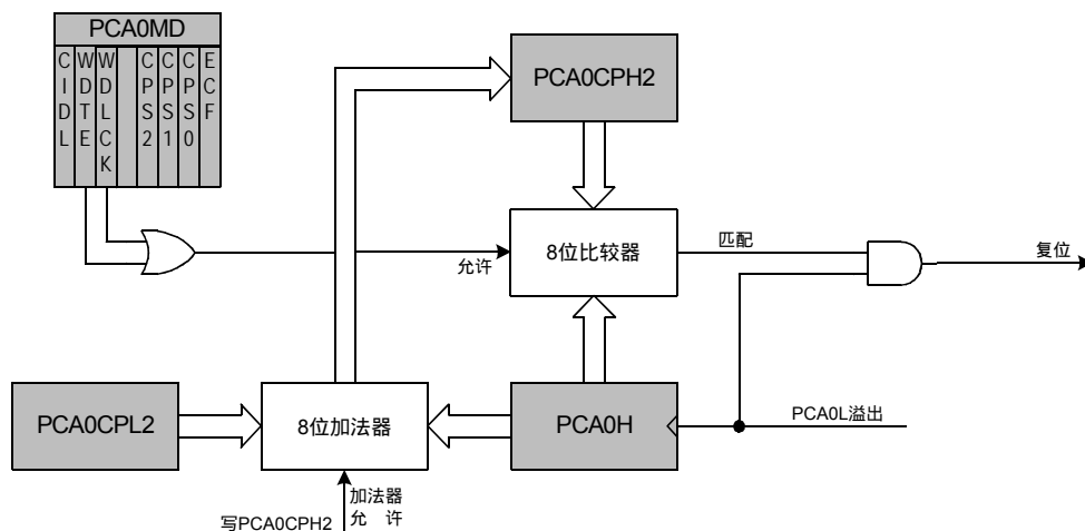
图 16.10 PCA 模块 2 的看门狗定时器方式
