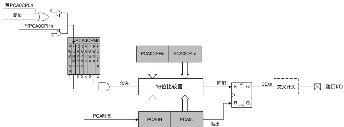
图 17.9 PCA 的 16 位 PWM 方式原理框图
