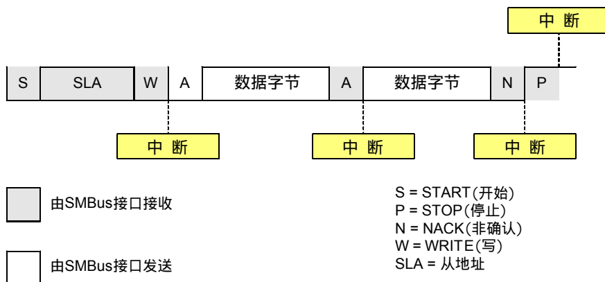
图 13.11 典型的从发送器时序
