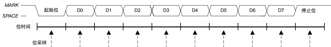
图 14.4 8 位 UART 时序图
