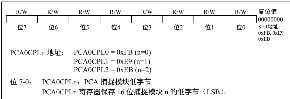
图 16.16 PCA0CPLn: PCA 捕捉模块低字节
