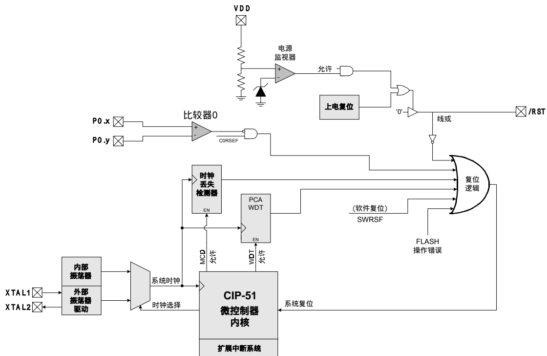
图 9.1 复位源框图
