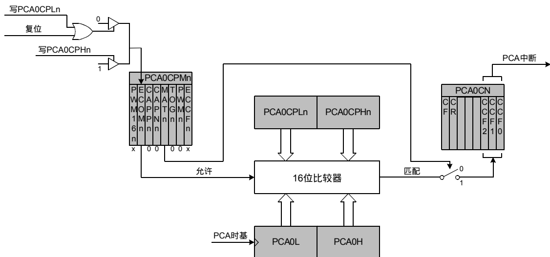
图 16.5 PCA 软件定时器方式原理框图
