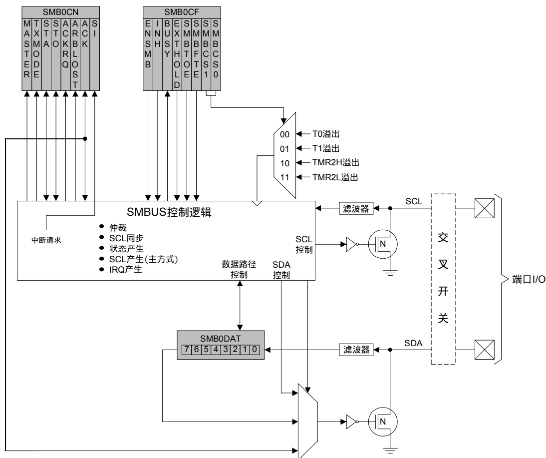
图 13.1 SMBus 原理框图
