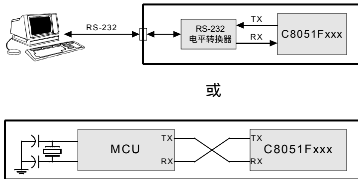
图 14.3 UART 连接图
