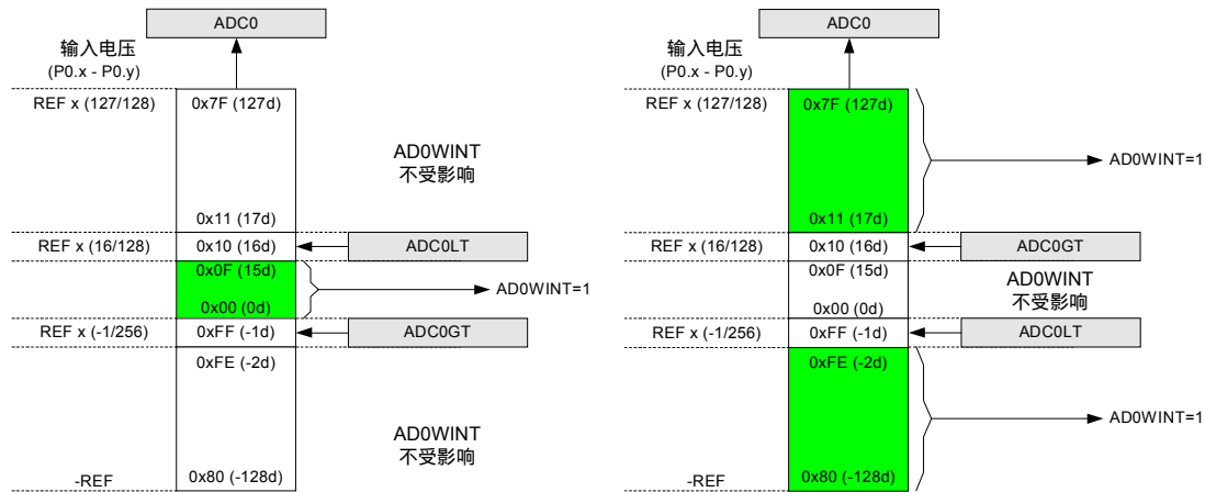
图 7.10 ADC 窗口中断示例（差分方式）
