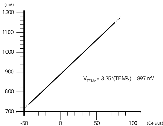
图 5.2 温度传感器典型传输函数
