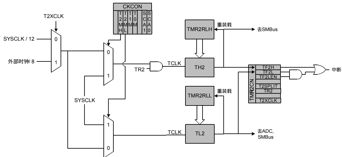
图 15.12 T2 方式 2 原理框图
