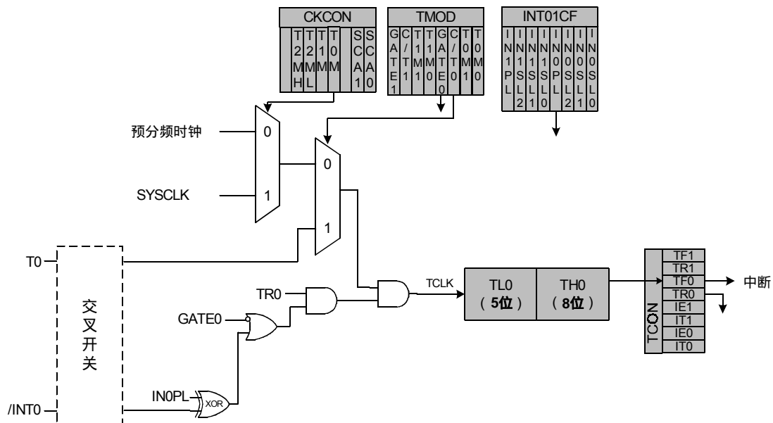
图 15.1 T0 方式 0 原理框图
