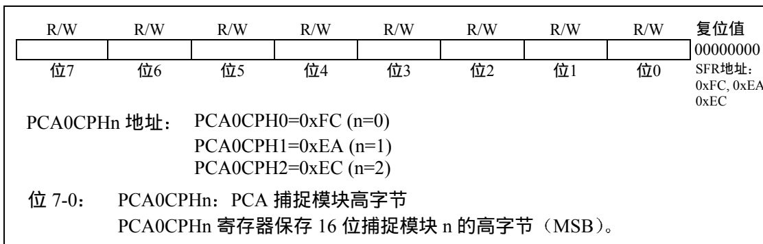
图 16.17 PCA0CPHn: PCA 捕捉模块高字节
