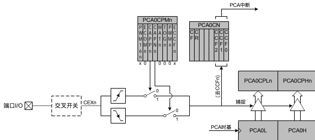
图16.4 PCA捕捉方式原理框图
