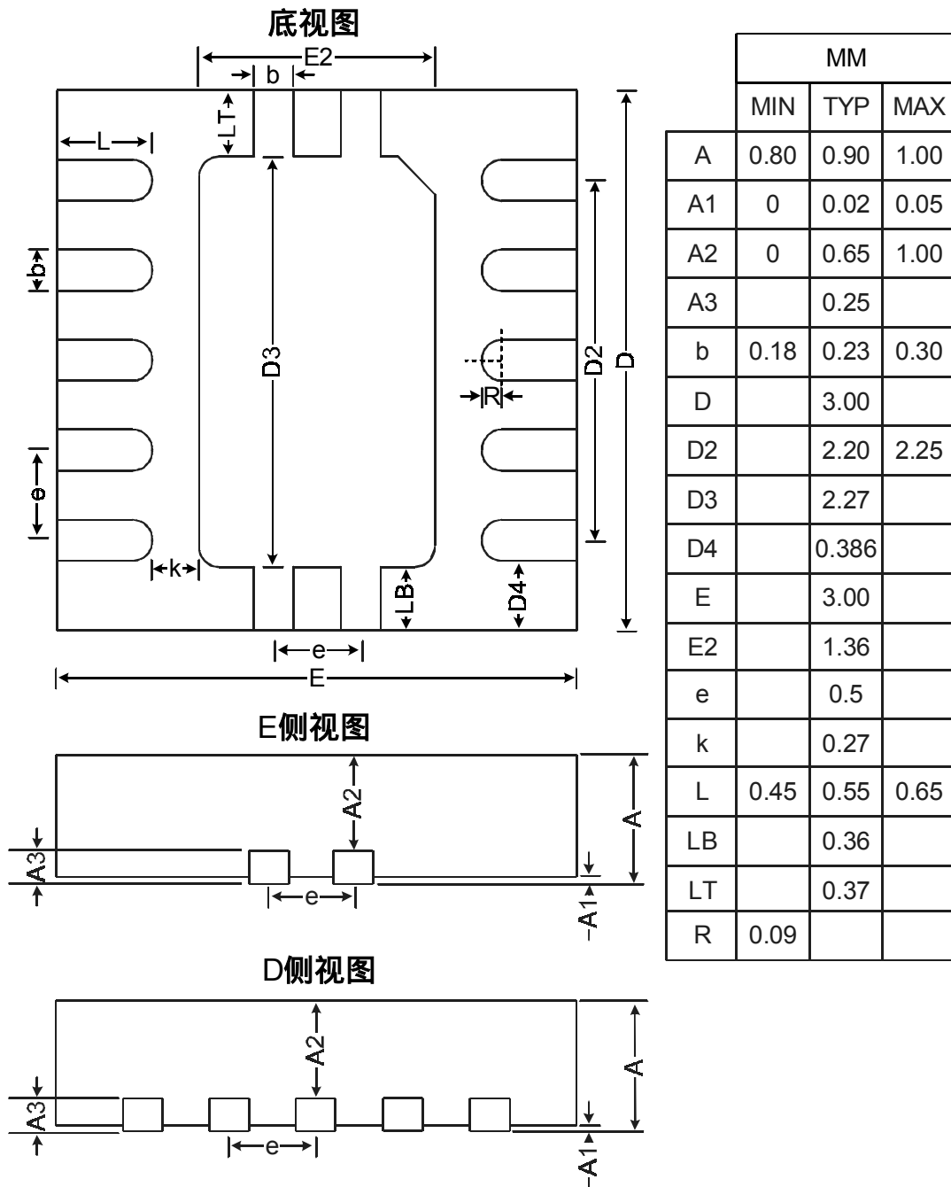
图 4.2 MLP-11 封装图
