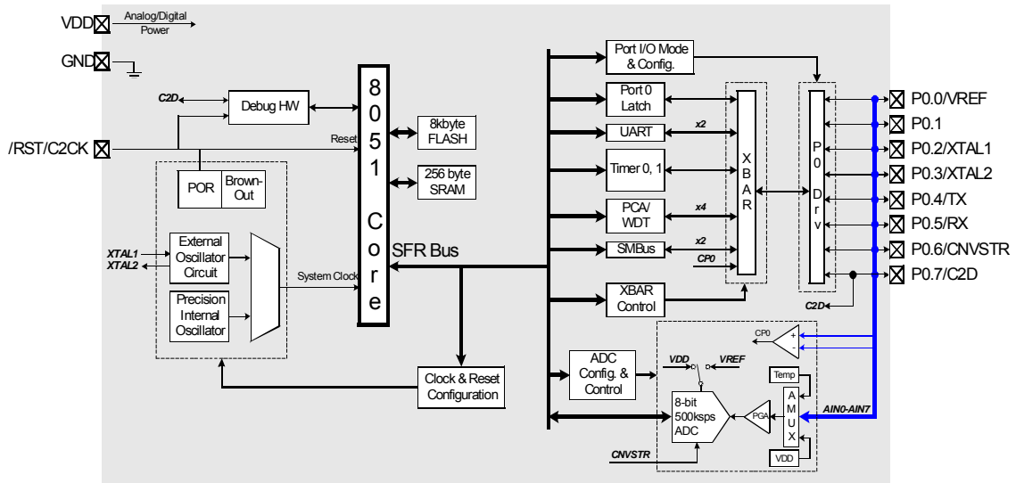
图 1.1 C8051F300/2 原理框图
