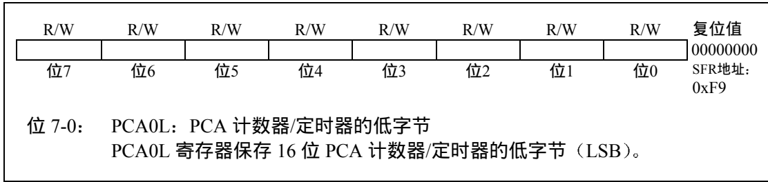
图 16.14 PCA0L: PCA 计数器 / 定时器低字节
