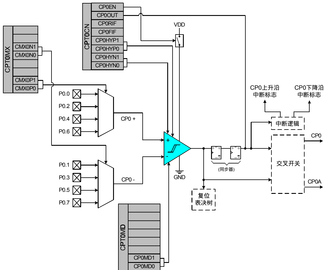
图 17.1 比较器功能框图
