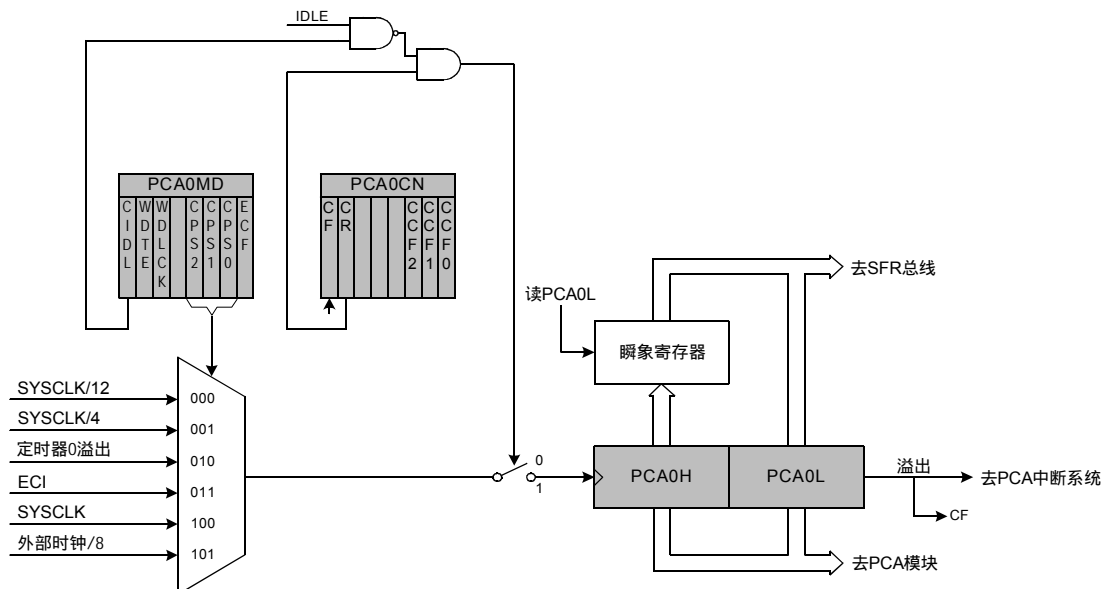
图 16.2 PCA 计数器/定时器原理框图
