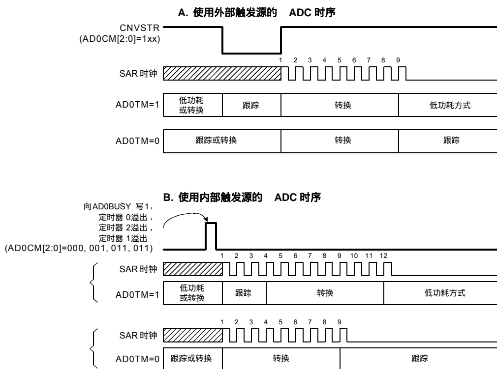
图 5.4 8 位 ADC 跟踪和转换时序示例
