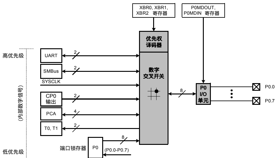
图 12.1 端口 I/O 功能框图
