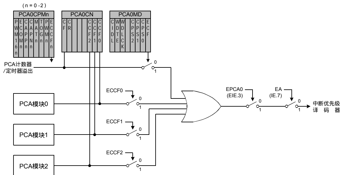
图 16.3 PCA 中断原理框图
