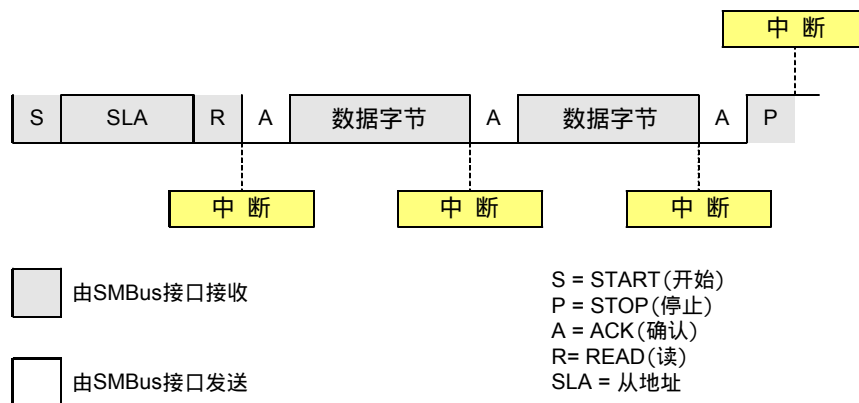
图 13.10 典型的从接收器时序
