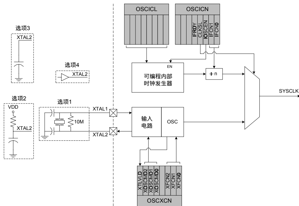
图 11.1 振荡器框图
