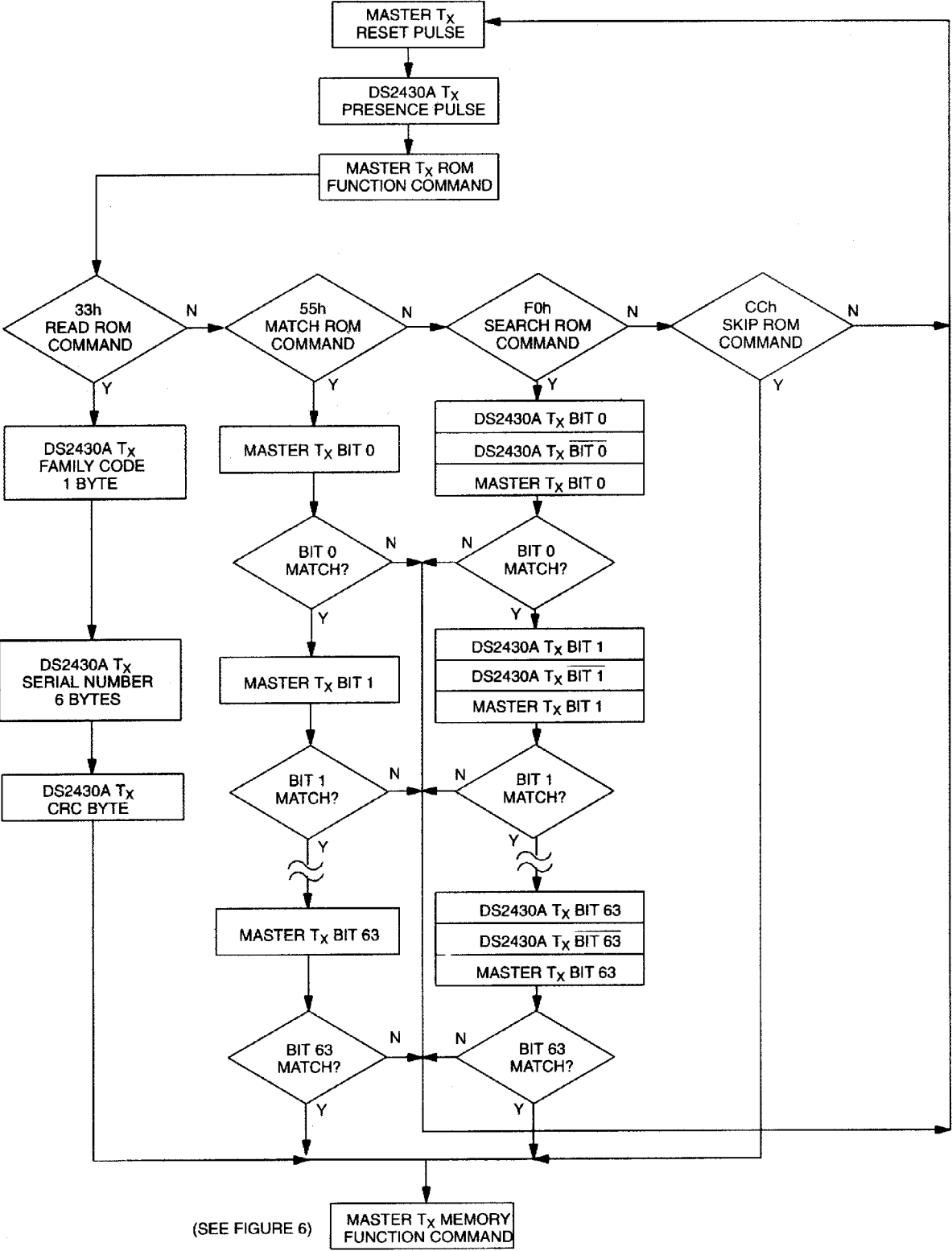
ROM 功能流程图 图 8
