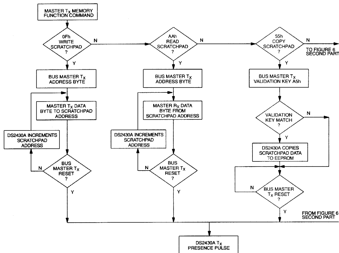
存储器功能流程图 图 6
