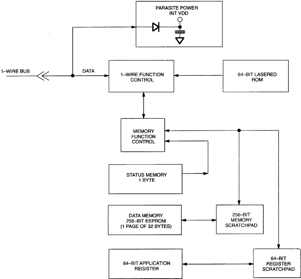
DS2430A 的内部框图 图 1
