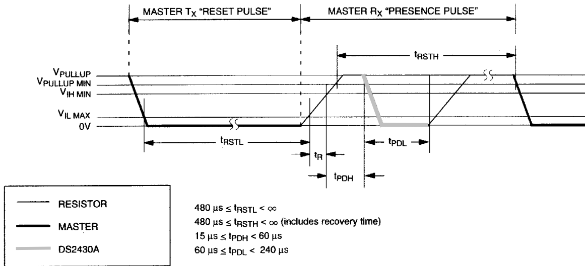
复位和应答脉冲的初始化时序 图 9
