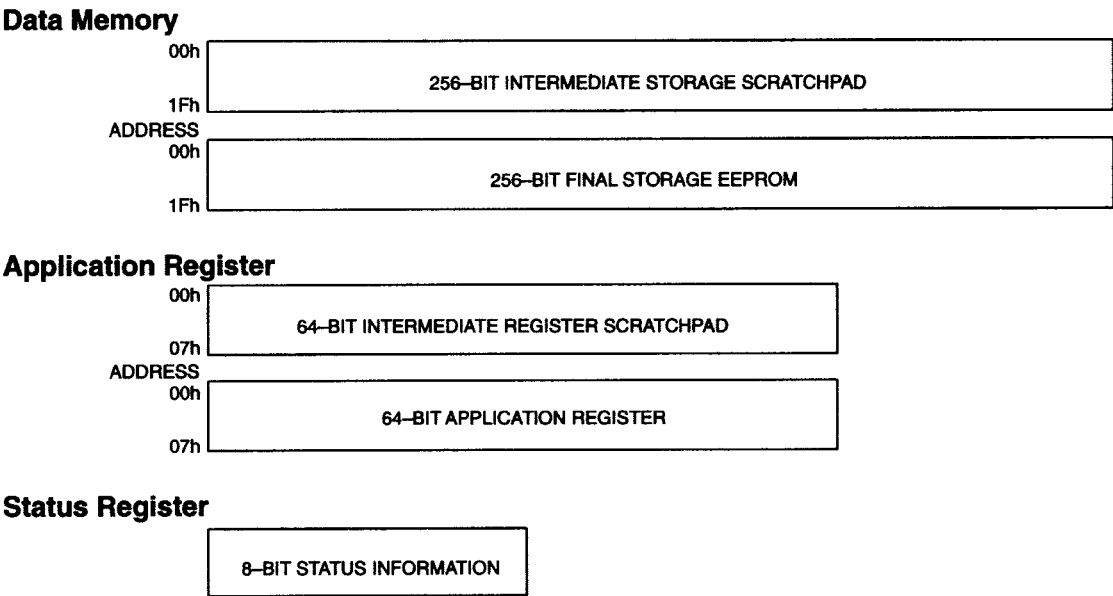
DS2430A 的存储器映射图 图 5
