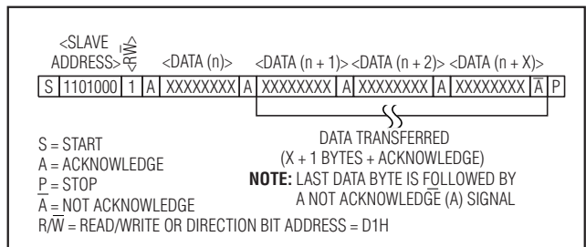
图4. 从设备发送模式 (读模式)
