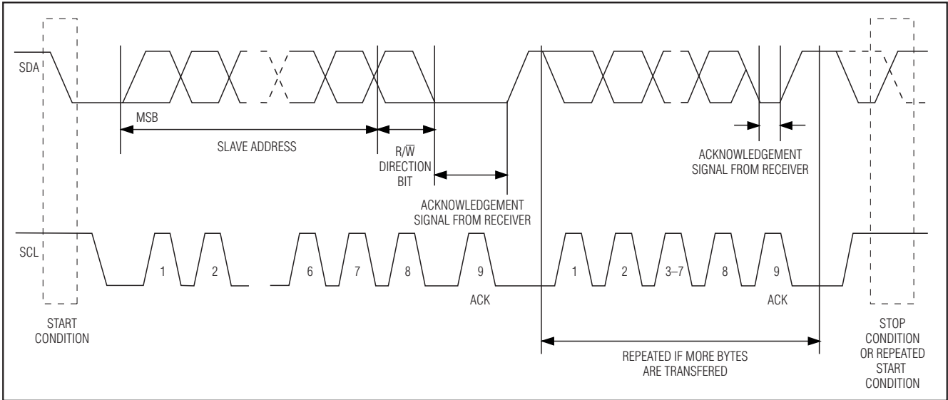
图2. I 2 C 数据传输示意图
