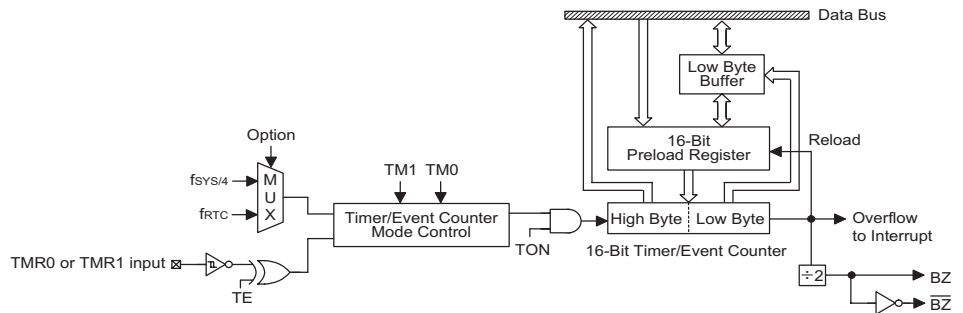
16 位定时/计数器结构
