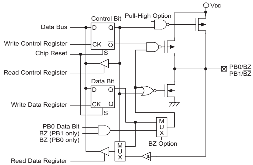
PB0/PB1 输入/输出端口
