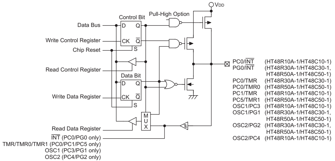
PB2~PB7、PC、PD、PE、PF 和 PG 输入/输出端口
