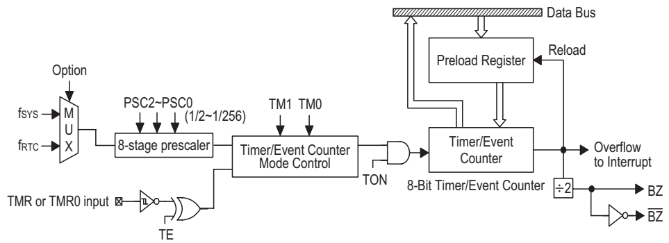
8 位定时/计数器结构
