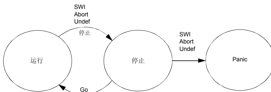
图 50 作为状态机的 RealMonitor
