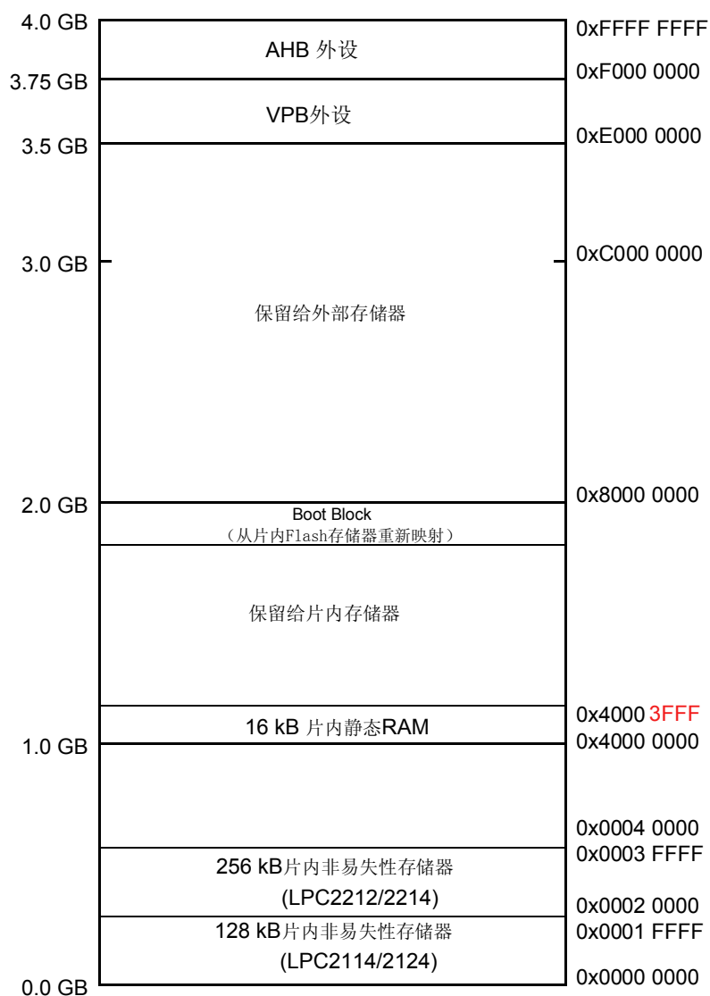
图2 系统存储器映射
