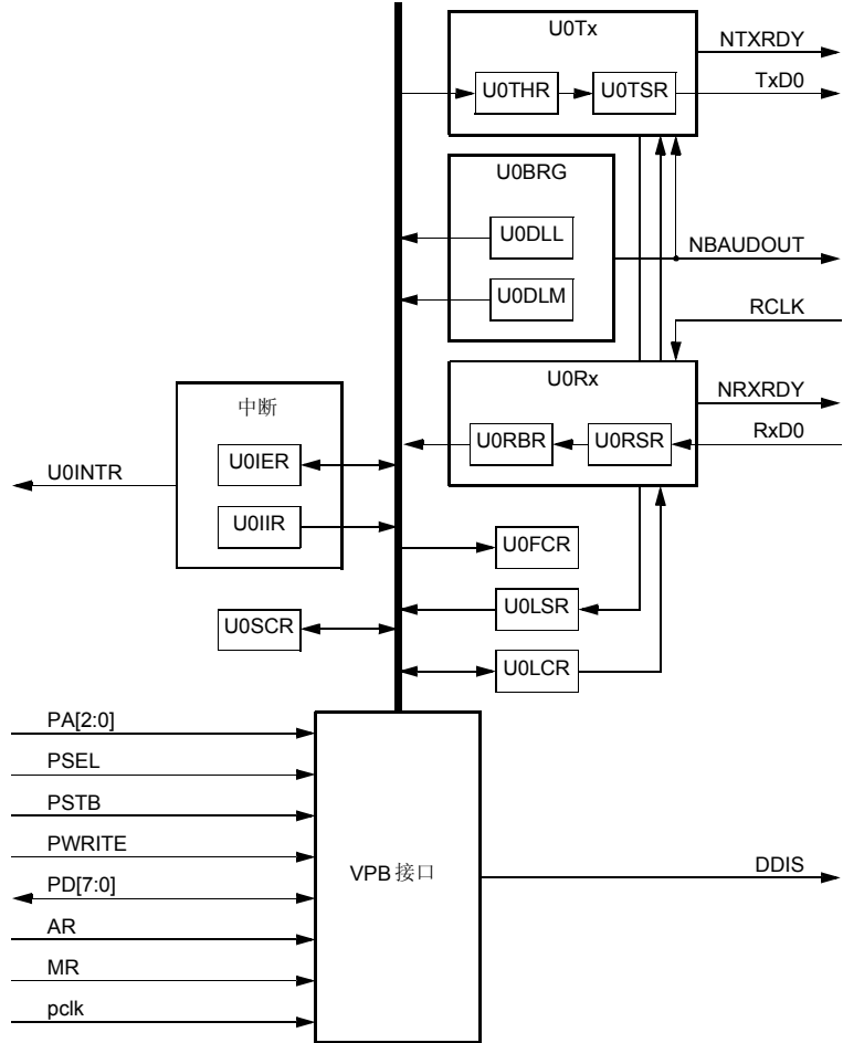
图 22 UART0 方框图
