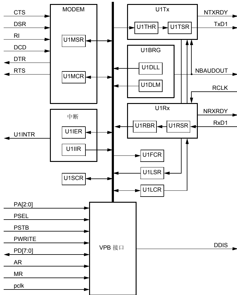
图 23 UART1 方框图
