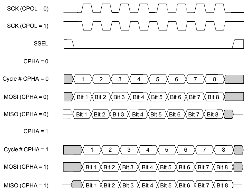
图 33 SPI 数据传输格式（CPHA=0 和 CPHA=1）
