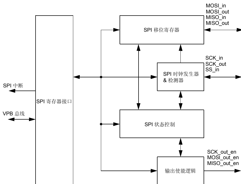
图 34 SPI 方框图
