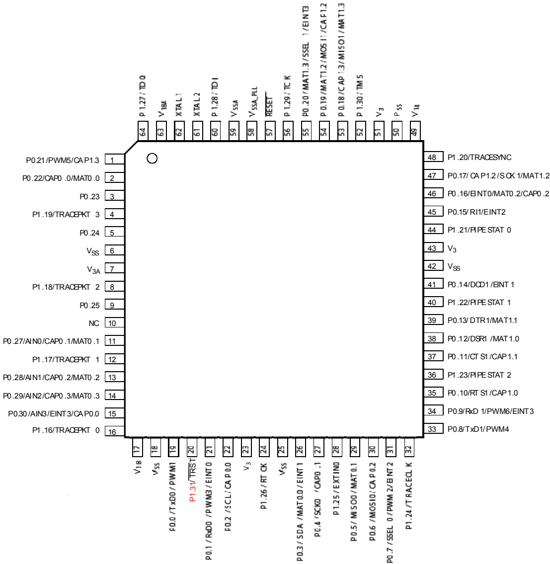
图 20 LPC2114/2124 的 64 脚封装
