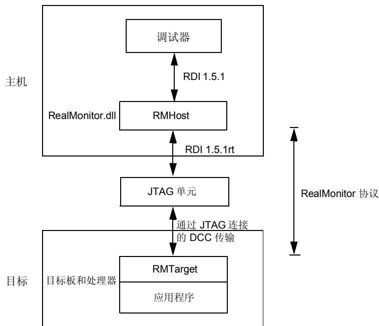
图 49 RealMonitor 部件
