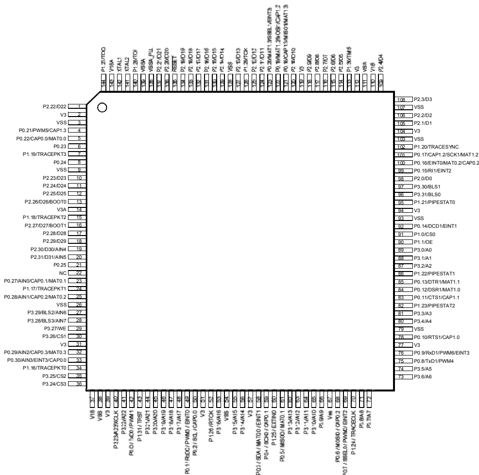
图 21 LPC2212/2214 的 144 脚封装
