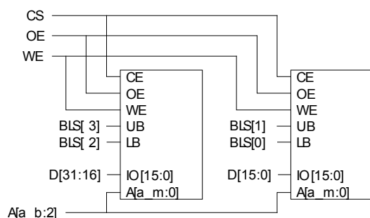
b) 32位宽存储器组连接16位的存储器芯片
