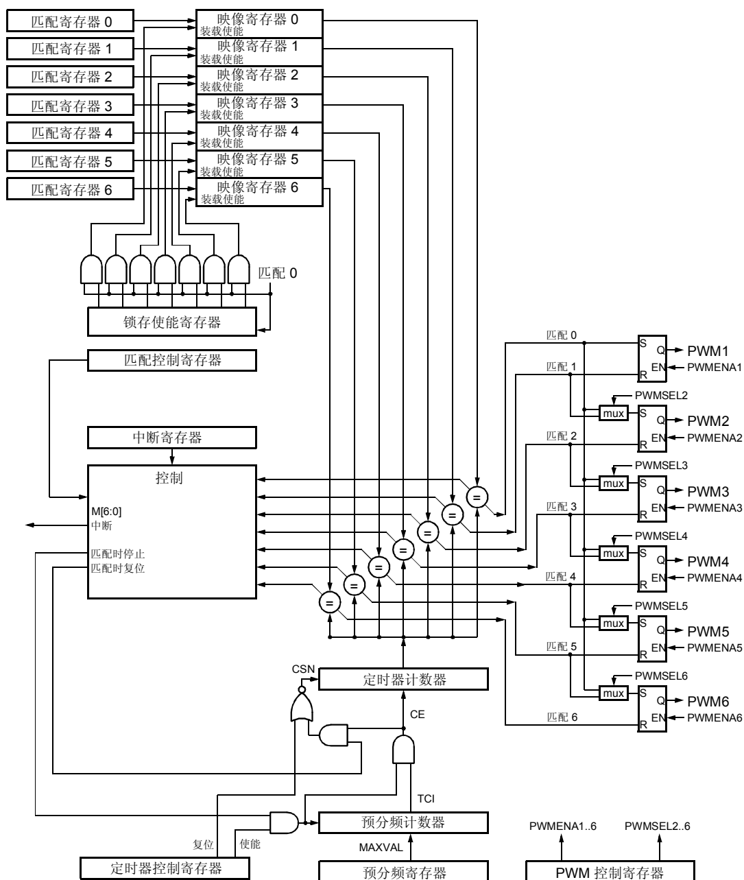
图 38 PWM 方框图
