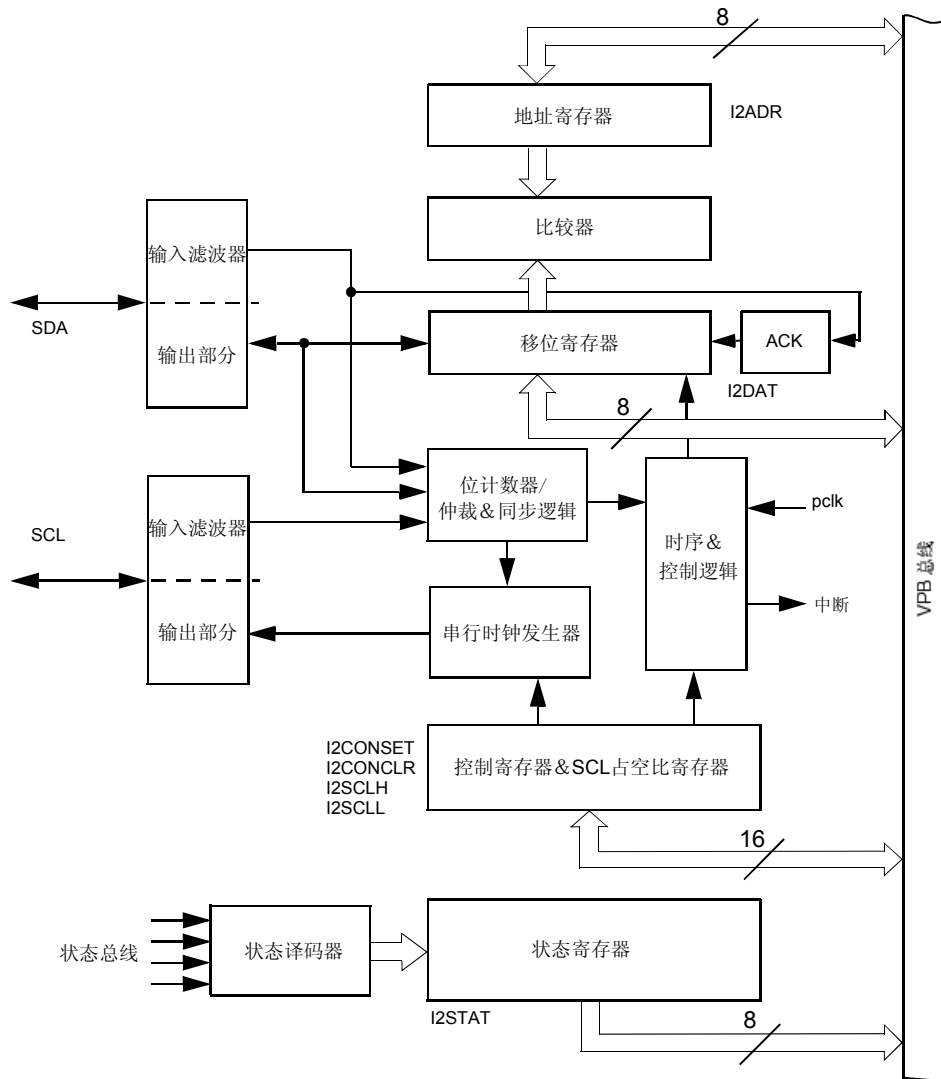
图 32 I 2 C 结构
