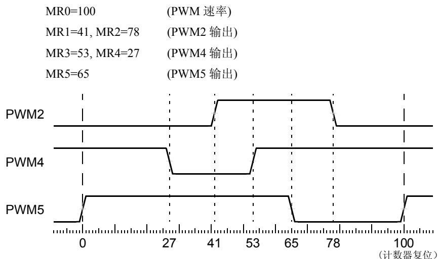
图 39 PWM 波形举例
