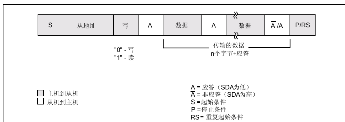
图 30 从接收器模式的格式
