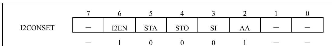
图 29 从模式配置
