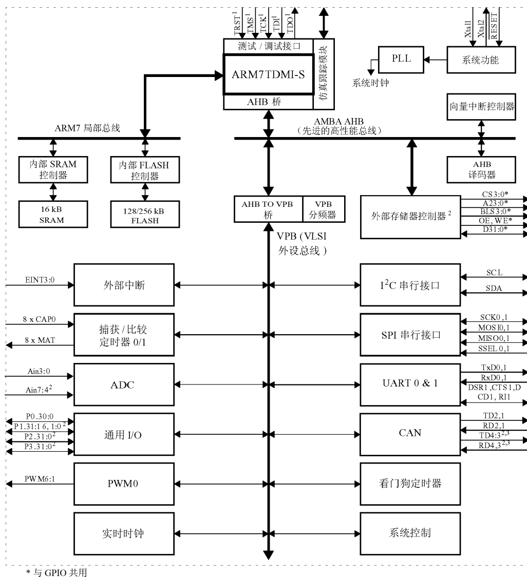
图 1 LPC2114/2124/2212/2214 方框图
