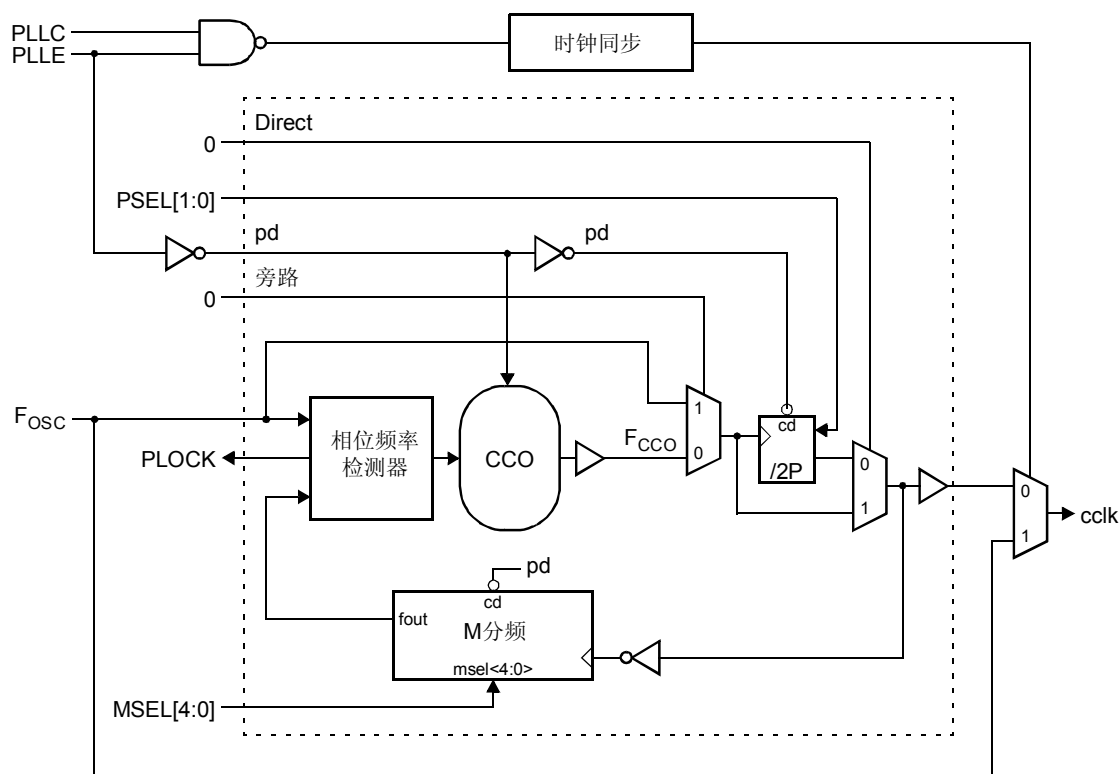
图 15 PLL 方框图
