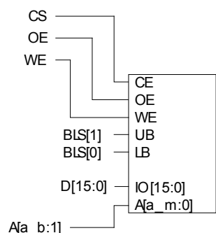
a) 16位宽存储器组连接16位的存储器芯片
