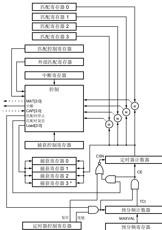
图 37 定时器方框图
