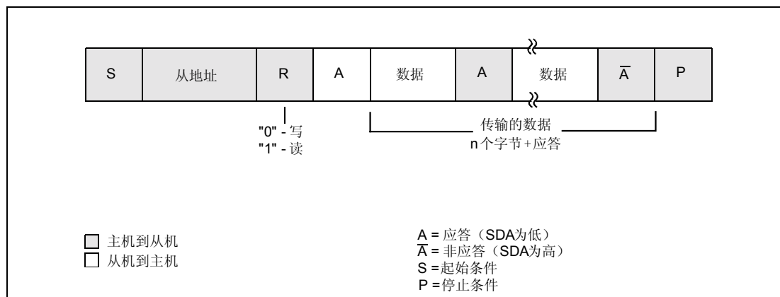
图 31 从发送器模式的格式
