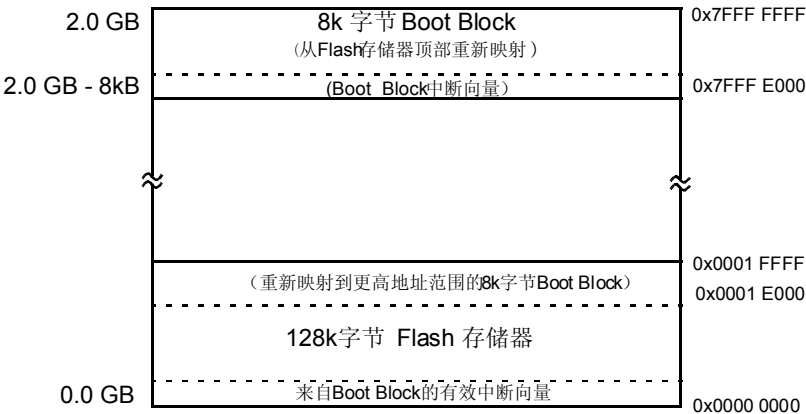
图 43 复位后低地址存储器的映射（128kB Flash 器件）
