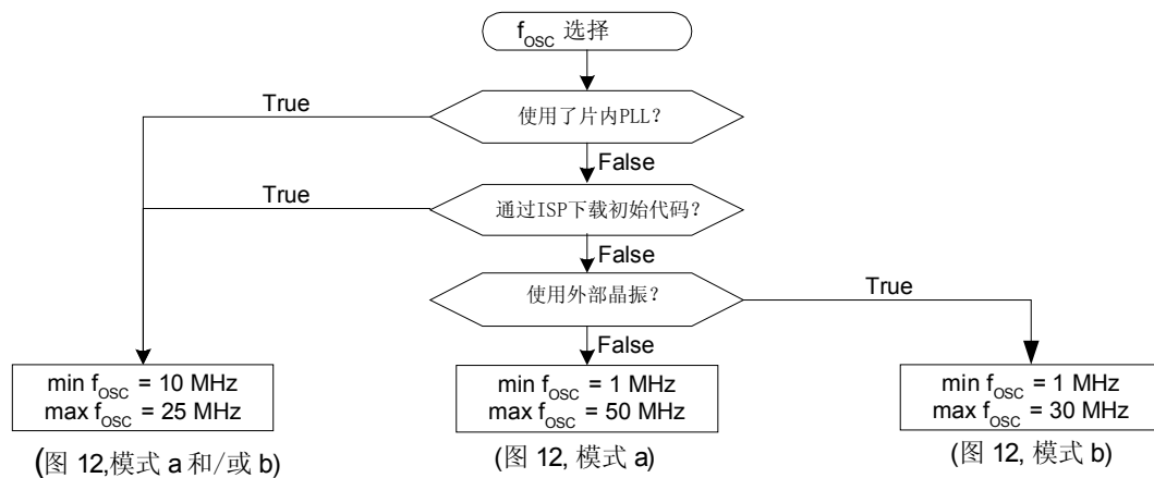
图 13 Fosc 的选择
