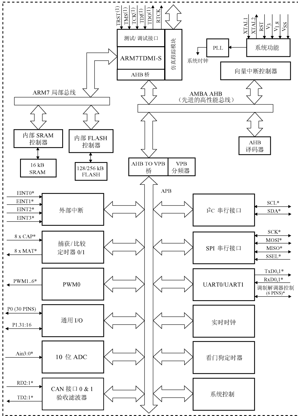
图 1 结构框图
