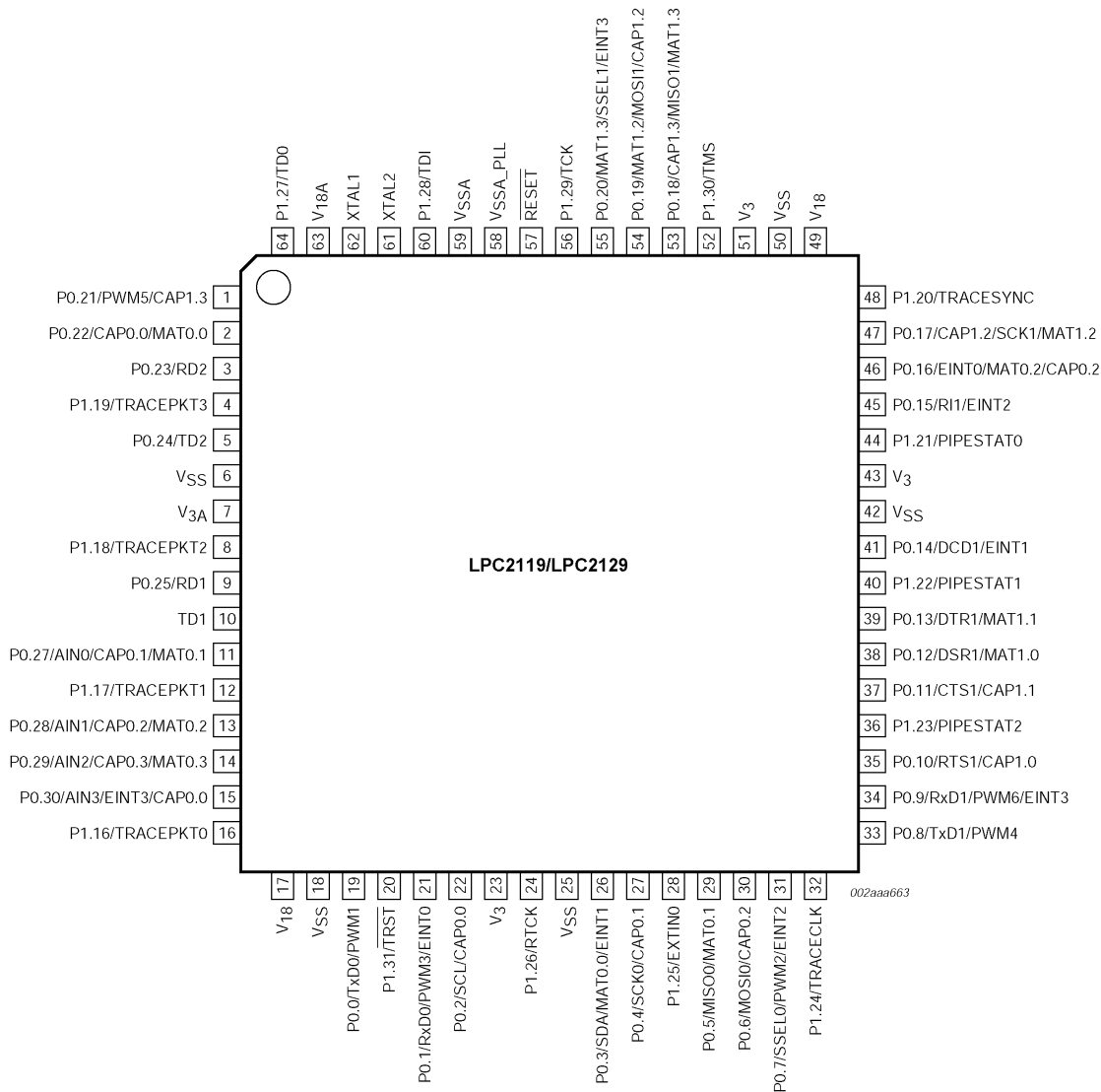
图 2 管脚排列
