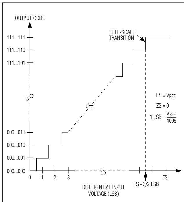
图8. 单极性传输函数 (仅适用于MAX1274)
