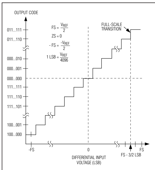
图9. 双极性传输函数 (仅适用于MAX1275)
