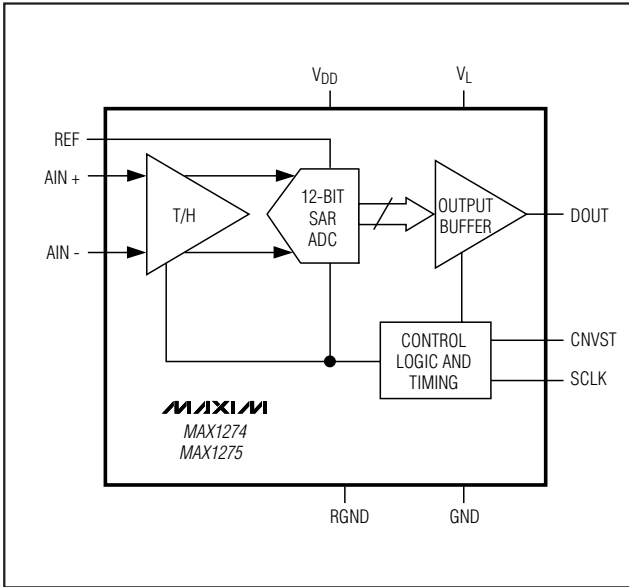
图3. 功能框图
