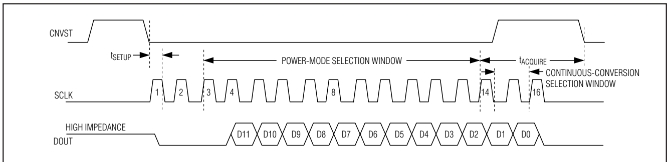
图5. 接口时序
