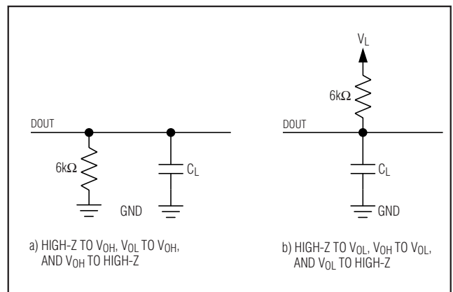
图2. 使能/禁用测试时间的负载电路
