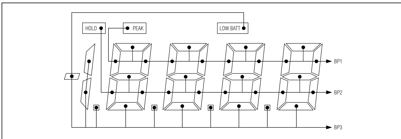
图4. MAX1494 (4位半) 背板连接图
