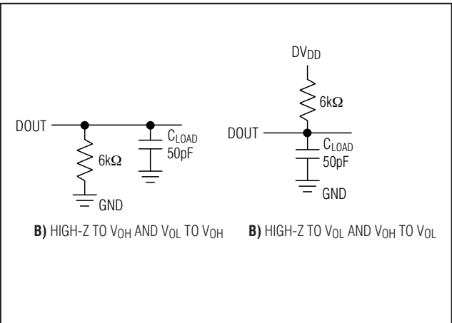
图19. 使能时间测试的负载电路
