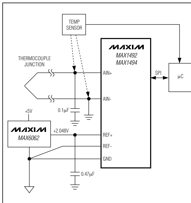
图21. MAX1492/MAX1494在热电偶系统的应用
