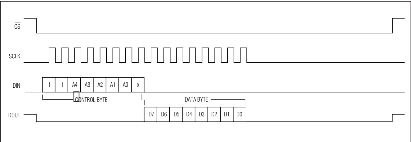
图17. 串口8位读操作时序图
