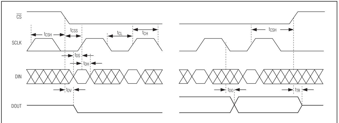
图13. 详细时序图
