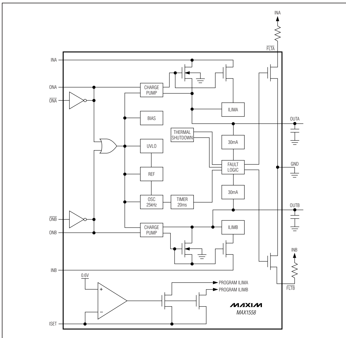
图 2. 功能框图
