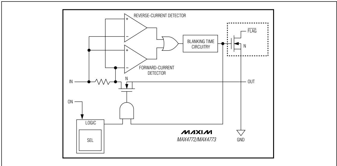
图1. 原理框图
