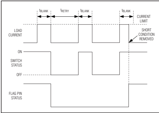
图4. MAX4773 自动重试故障屏蔽时序图
