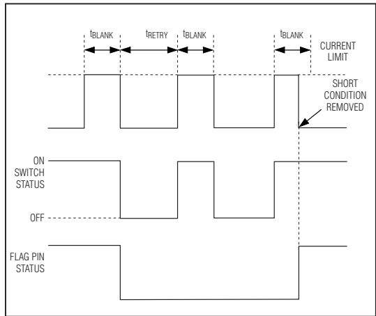
图2. MAX4796/MAX4798 自动重试故障屏蔽时序图
