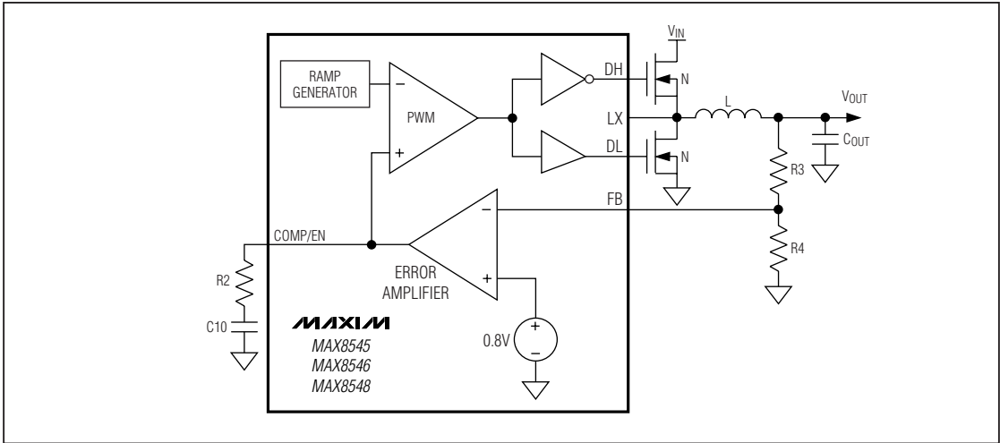
图3. 补偿原理
