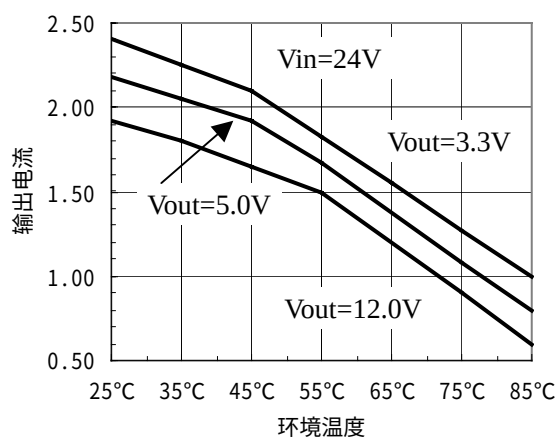
PSP200SRP 连续输出电流与环境温度
