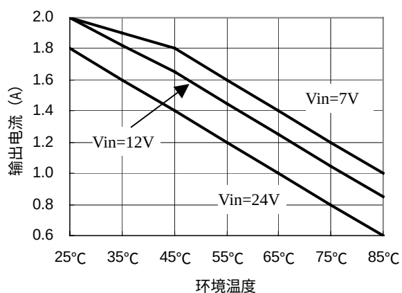
PSC210SRP-3.3 连续输出电流与环境温度
