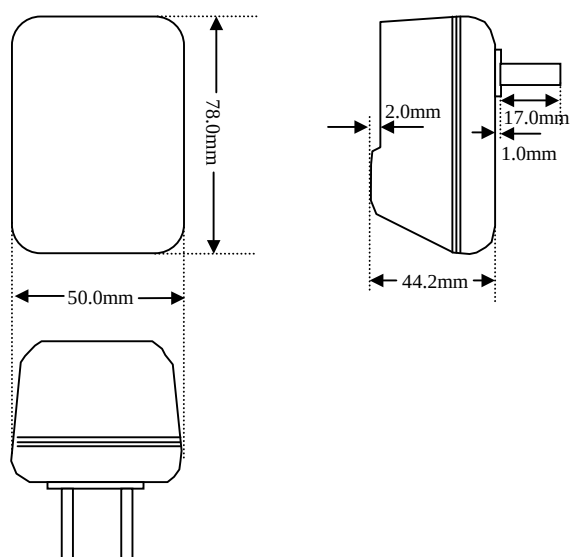
外置式 AC-DC 适配器外形尺寸图
