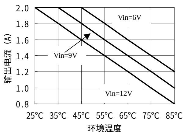
PSC200SRP-5.0 连续输出电流与环境温度
