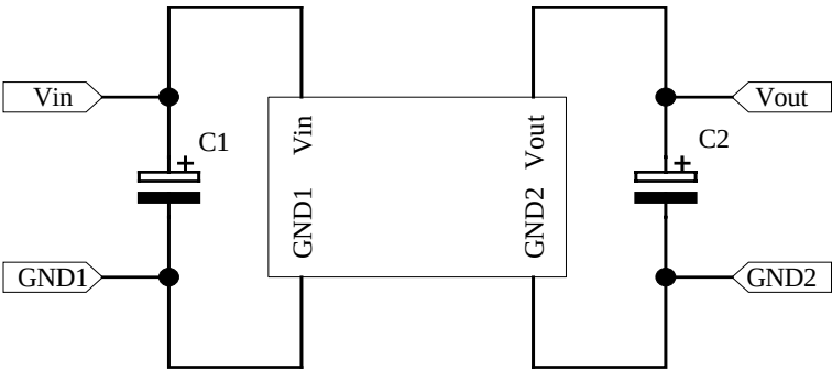
C1 按《产品性能指标及选购指南》选择，C2 是可选的滤波电容
