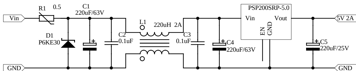
PSP200SRP-5.0 将 24V 车载电瓶电压变换成 5V 的参考应用电路
