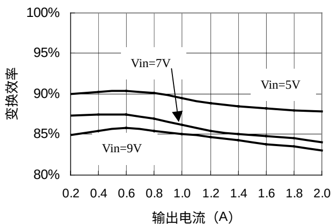
PSC200SRP-3.0 典型变换效率
