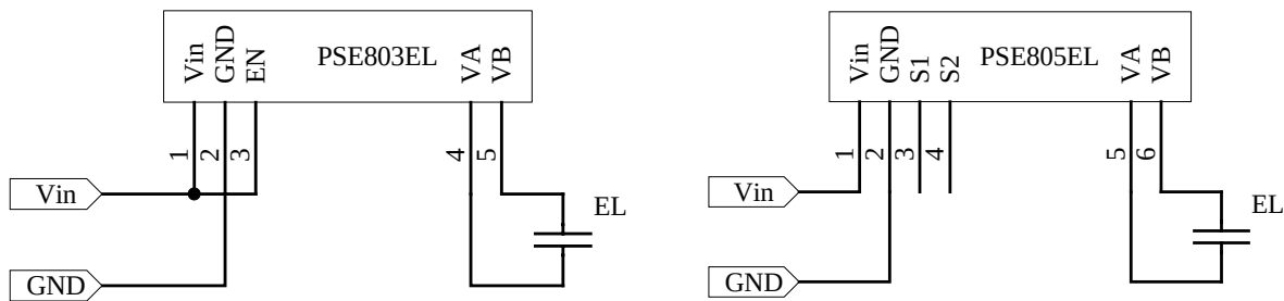
PSE803EL 典型应用电路
