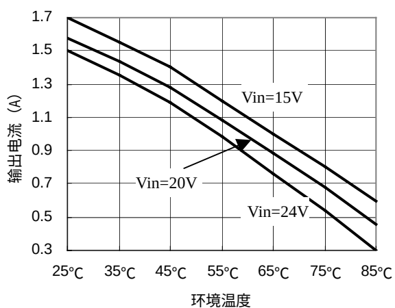
PSC210SRP-5.0 连续输出电流与环境温度
