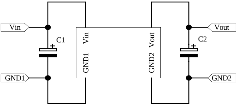
C1, C2 是可选的滤波电容
