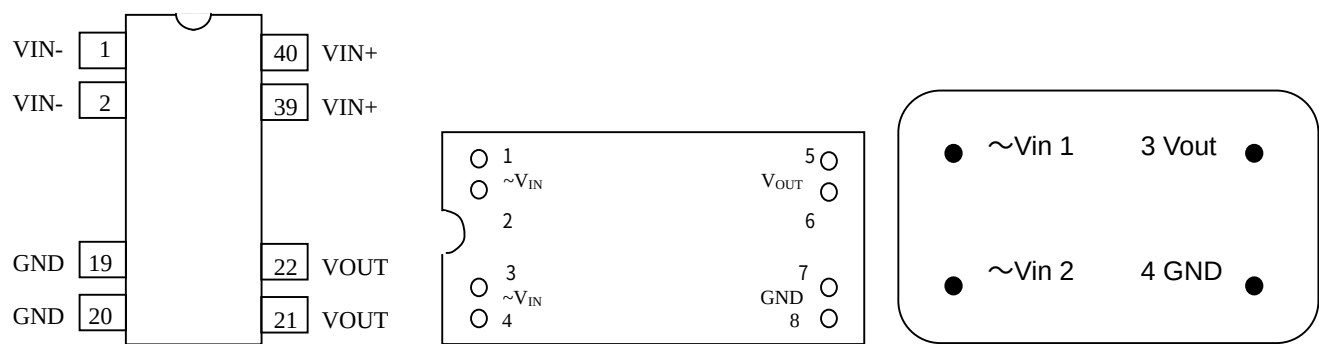
53x19 DIP40 电胶木 54x28 电胶木（顶视图） 68x45 金属铝（顶视图）
