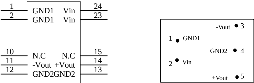
LDIP24 50.8x25.4 金属封装（顶视图）
