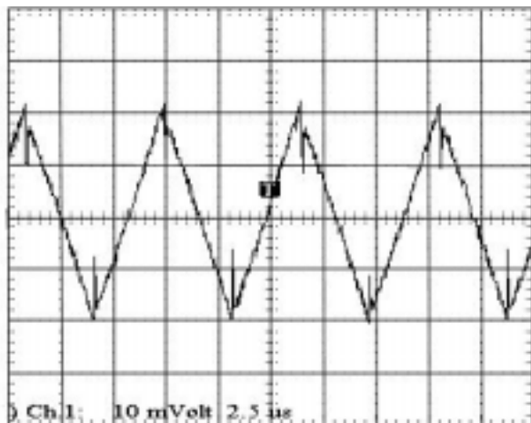
PSP100B-5.0 输出电压纹波 (工作条件: V_{in}=12V , V_{out}=5V , I_{out}=1A , T_a=25^{\circ}C )
