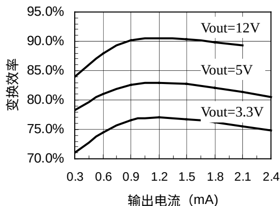
PSP200SRP 变换效率与负载电流关系
