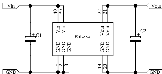
PSL 升压或降压系列典型应用电路（C1 为可选元件、C2 可选 100\mu\text{F}\sim 220\mu\text{F} ）
