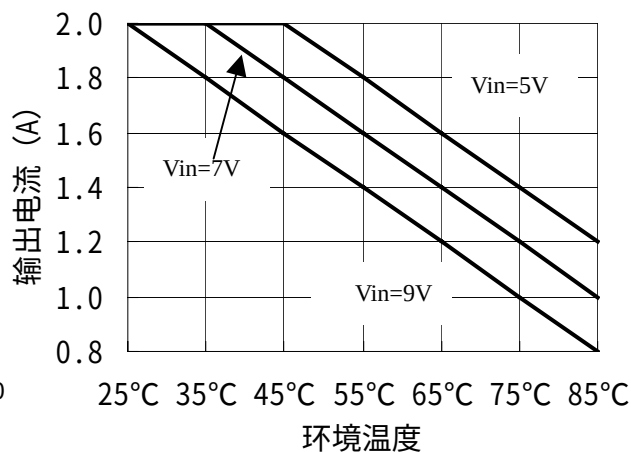
PSC200SRP-3.3/3.0 连续输出电流与环境温度
