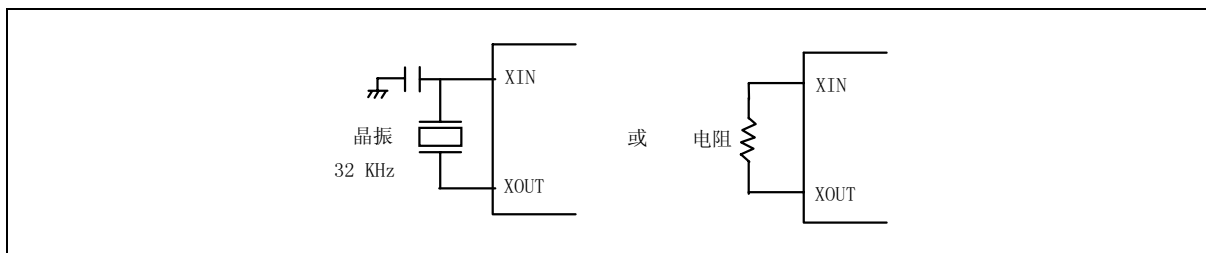
图3. 振荡器的配置
