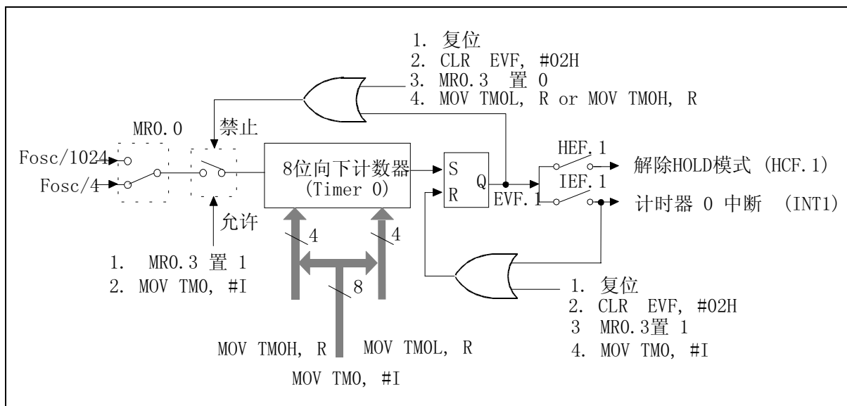
图6. 定时器0的结构
